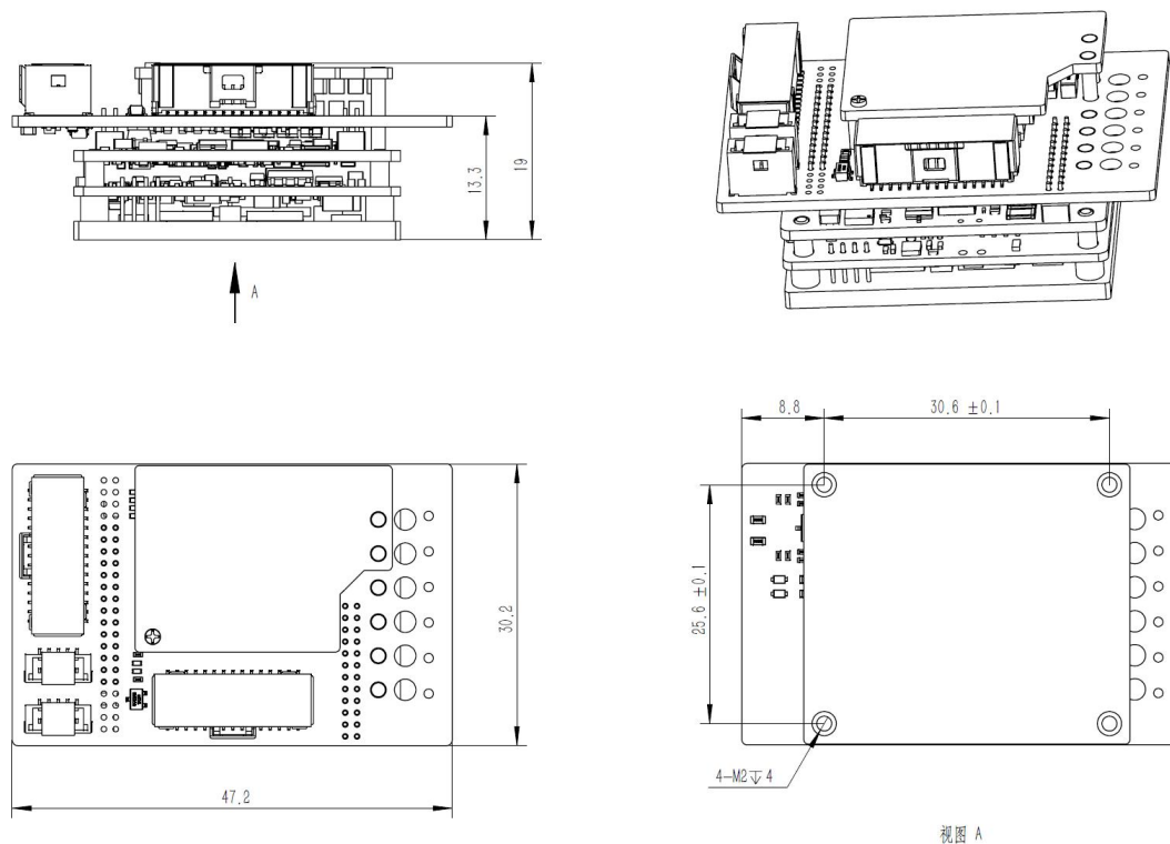
图 1-5 CANopen 版本驱动器安装图纸
