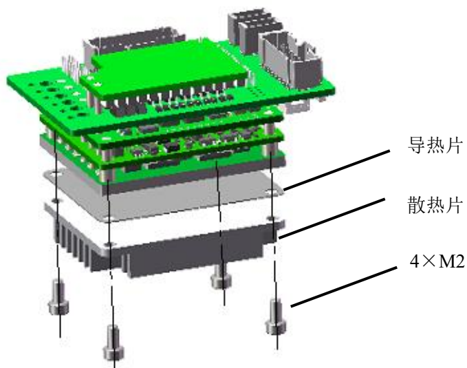
图 3-1 散热附件安装示意图
