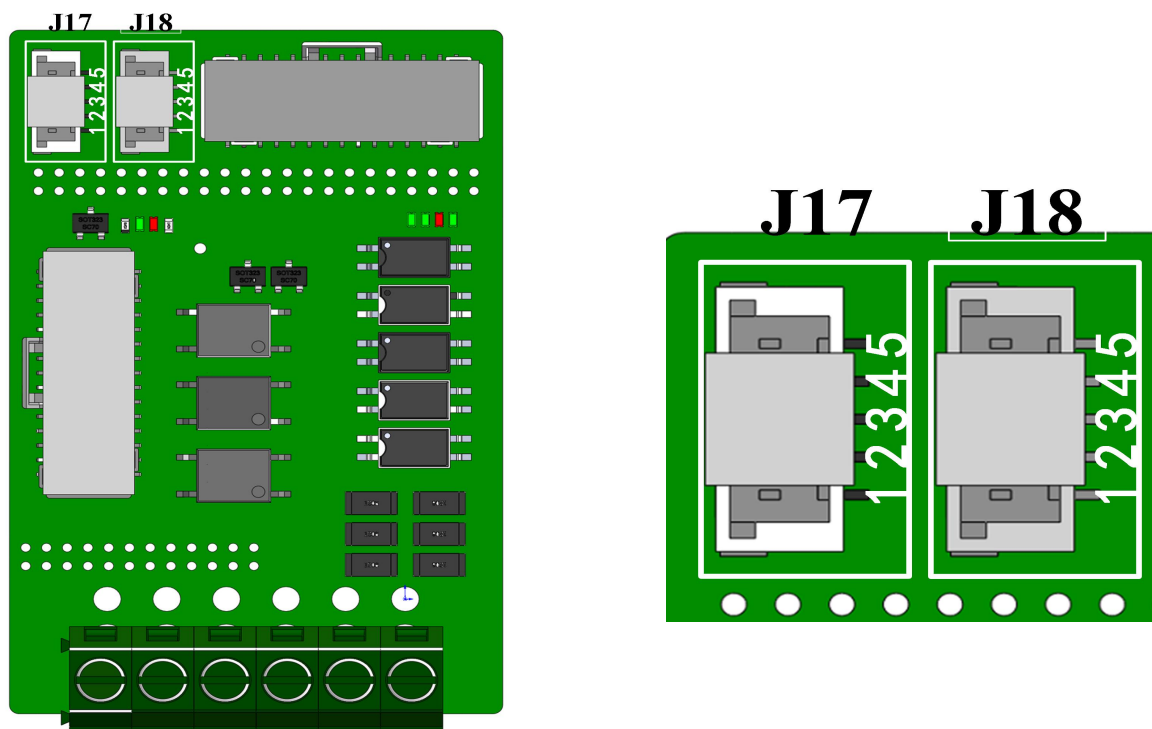
图 4-9 EtherCAT 通讯接口示意图
