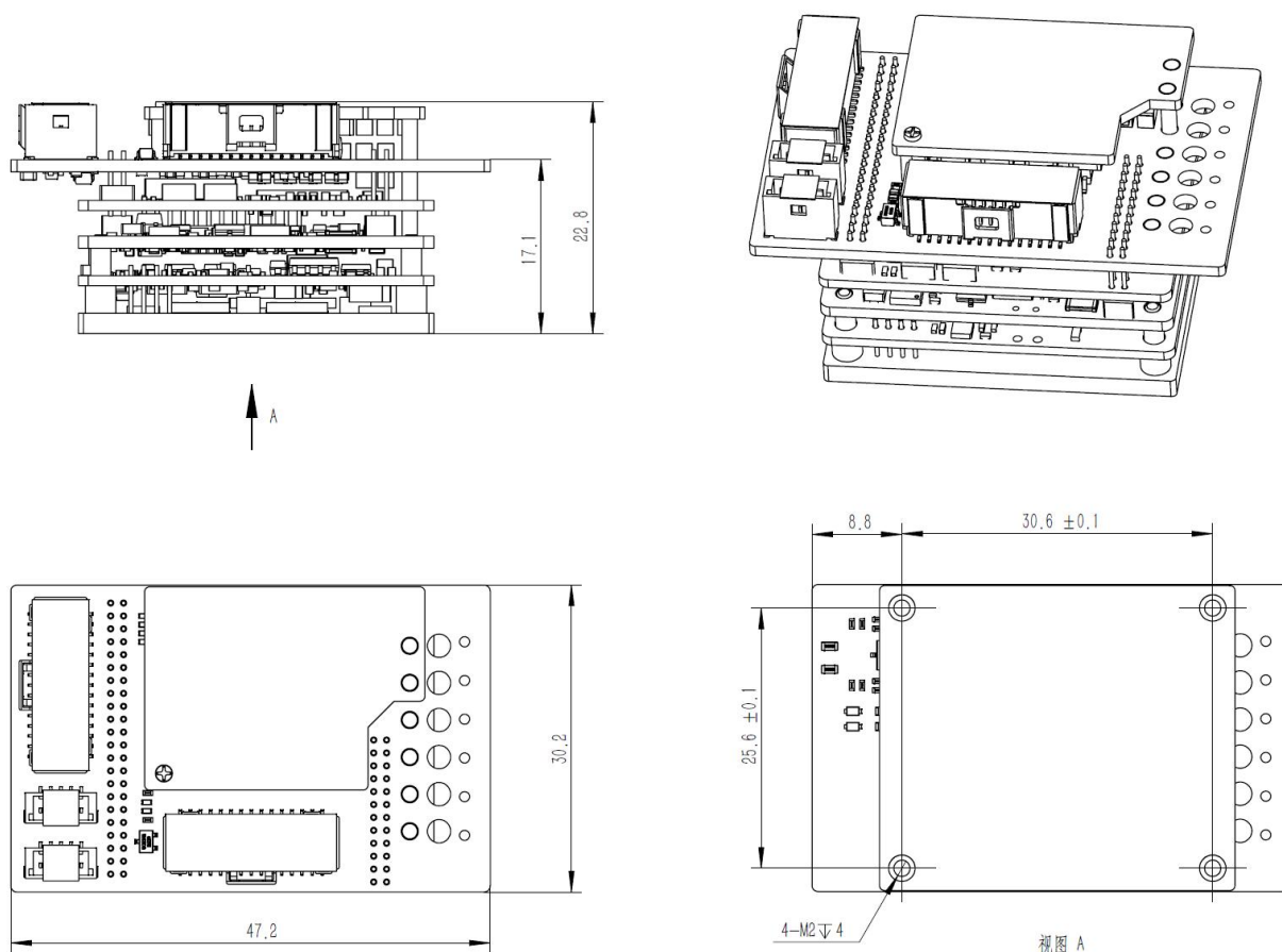
图 1-7 EtherCAT 版本驱动器安装图纸
