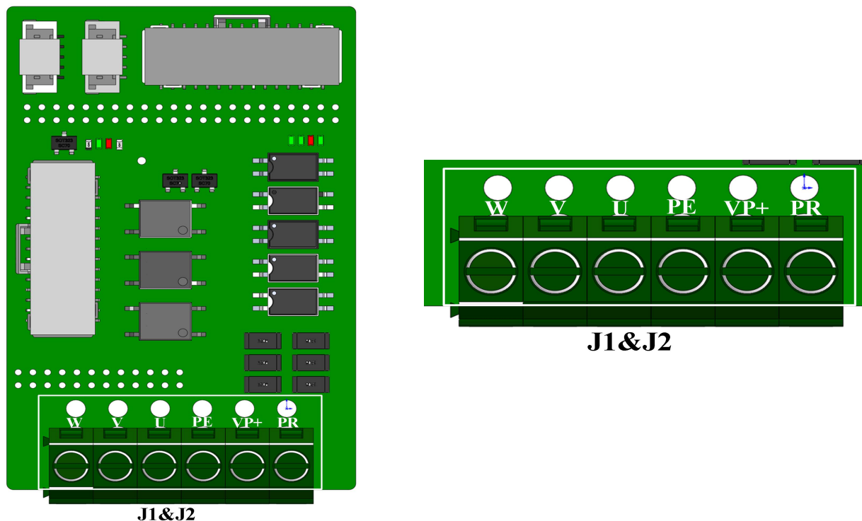
图 4-2 电源接口示意图
