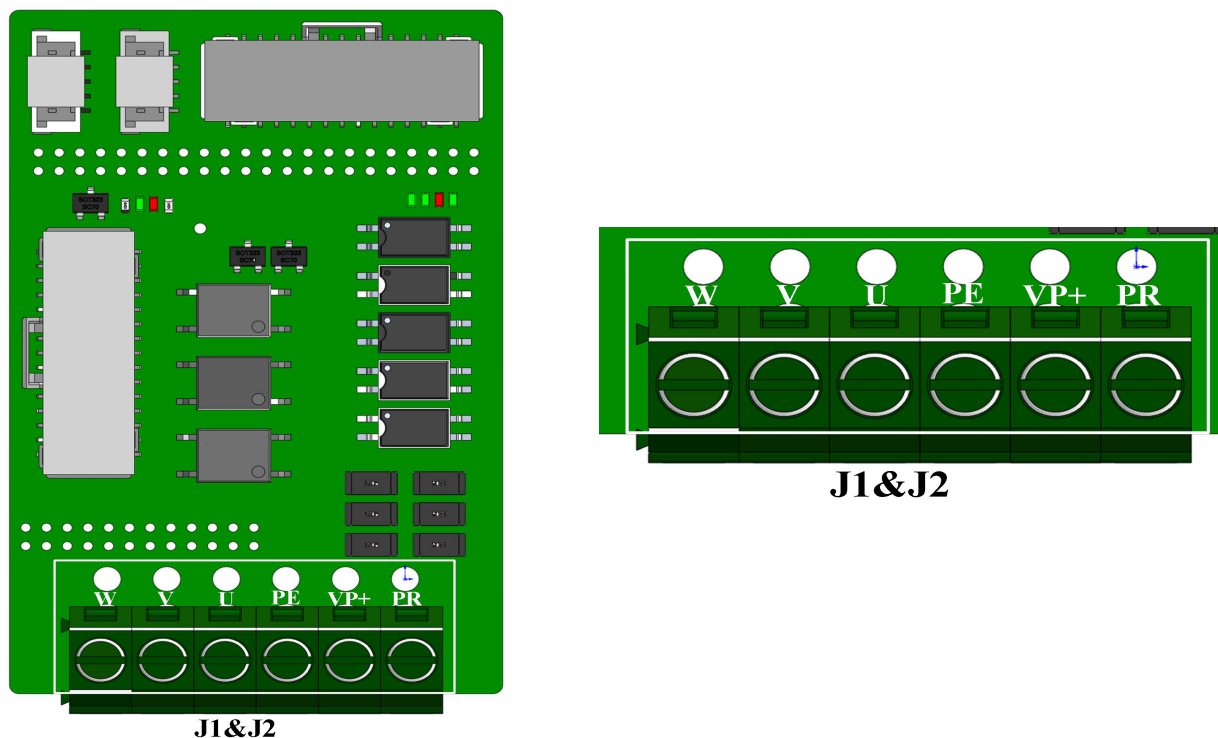
图 4-4 动力线接口示意图
