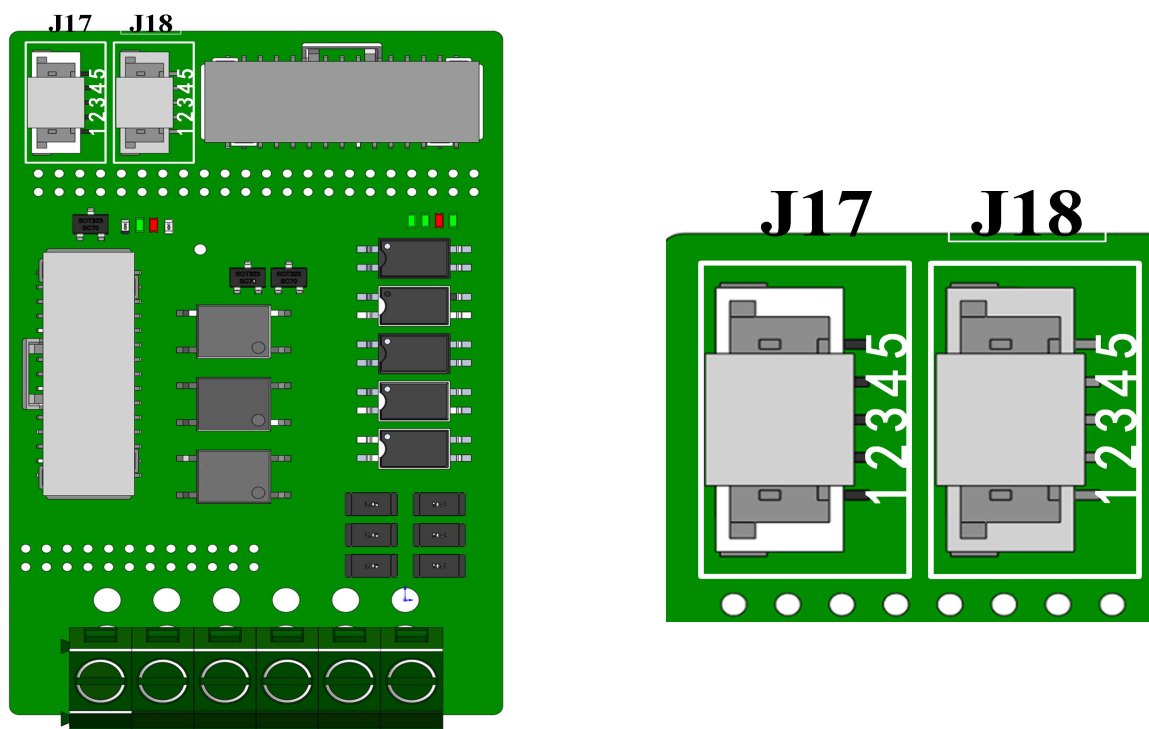
图 4-7 CAN/CAN FD 通讯接口示意图
