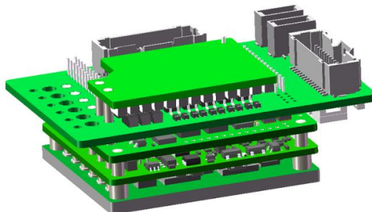
图 1-2 焊线驱动器外观图
