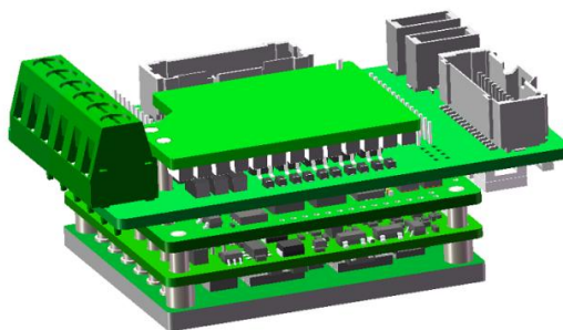
图 1-1 立式端子驱动器外观图
