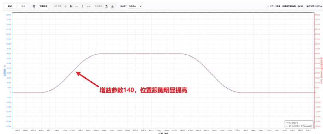
位置环增益 140
