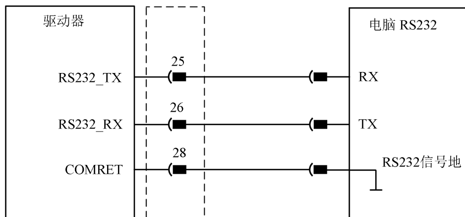
图 4-46 RS232 接线示意图
