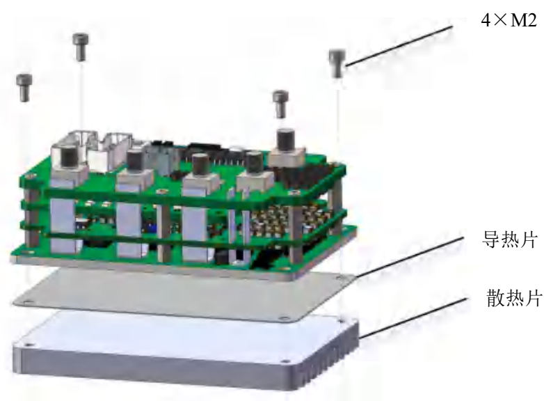
图 3-2 CANopen 版散热附件安装示意图
