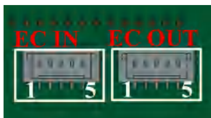
EtherCAT 版 100V 端子脚位示意
