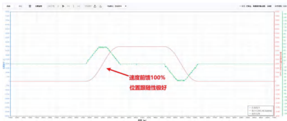
速度前馈 100%
