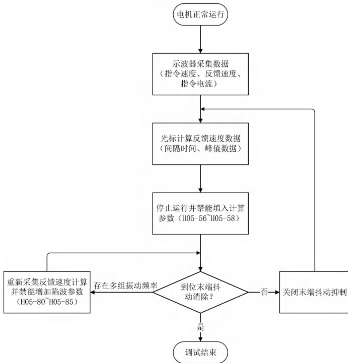
图 1-11 低频振动抑制操作流程圖
