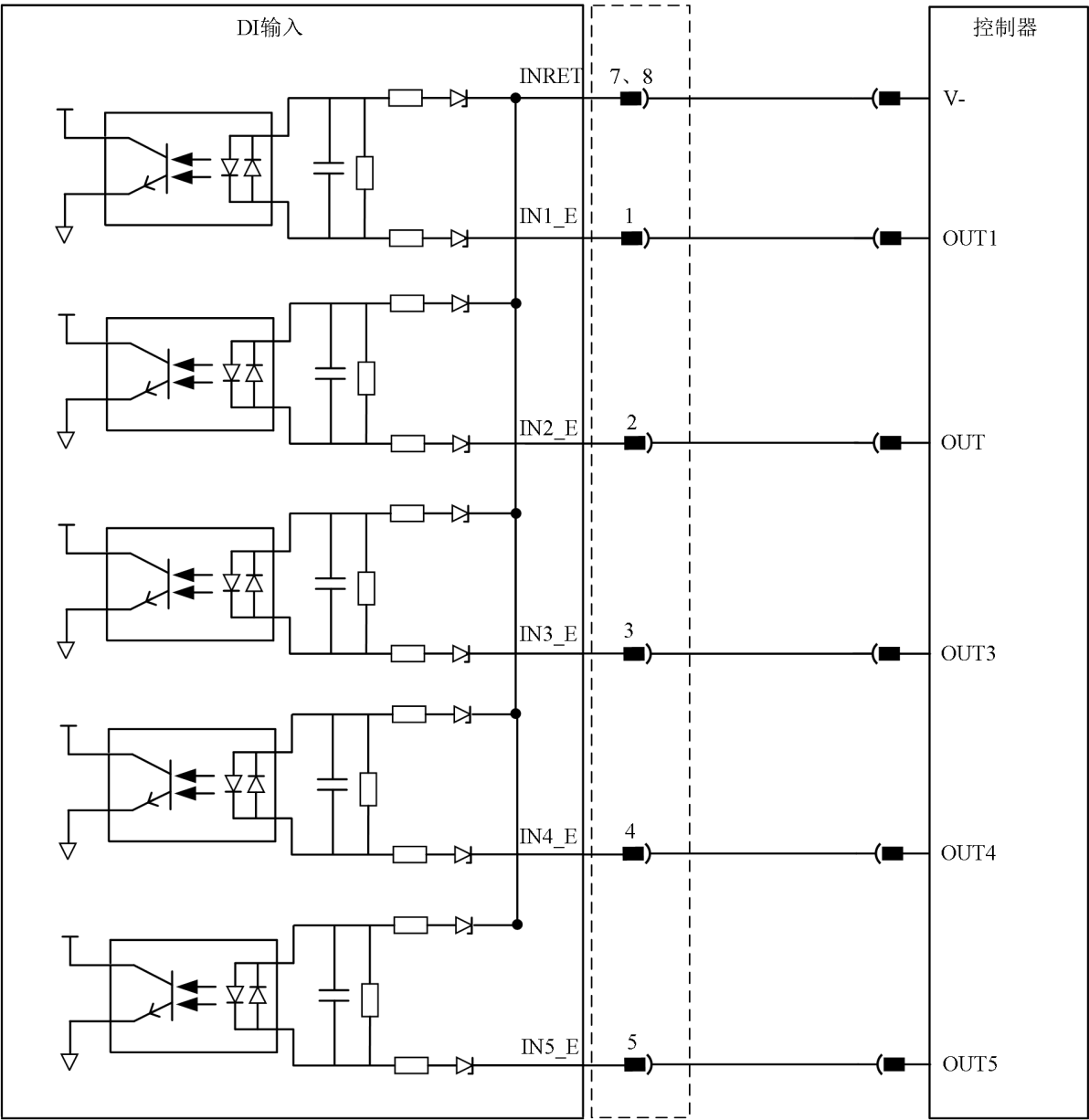
图 4-39 源型输入接线图
