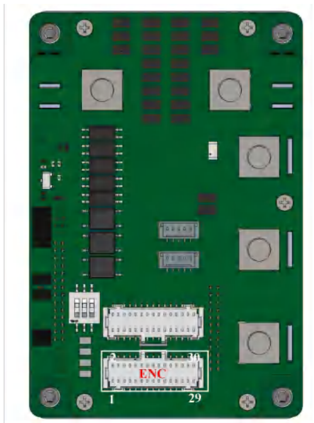
CAN 版 100V 端子脚位示意
