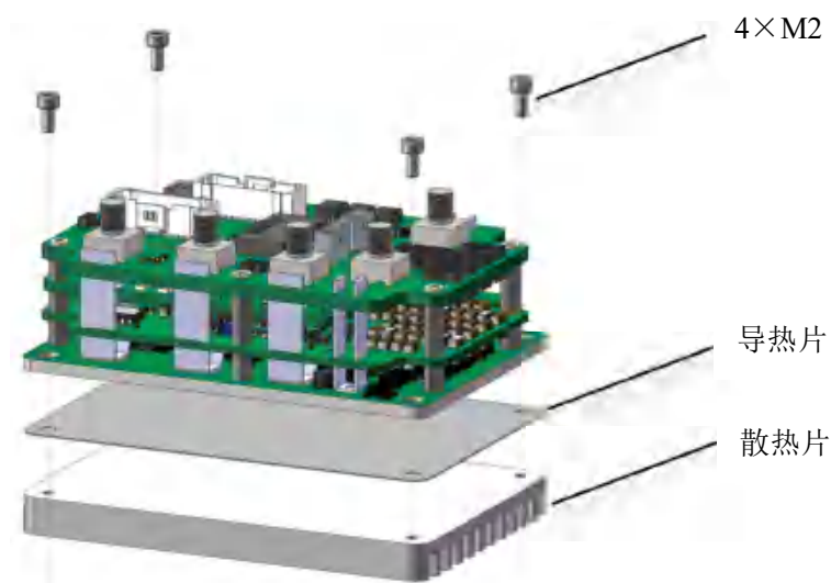
图 3-1 EtherCAT 版散热附件安装示意图
