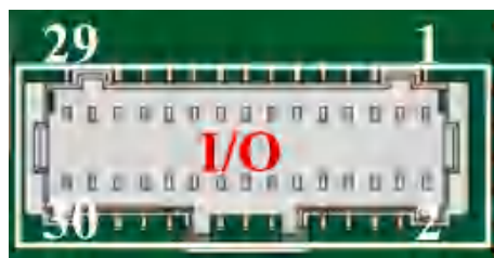
CAN 版 100V 端子脚位示意
