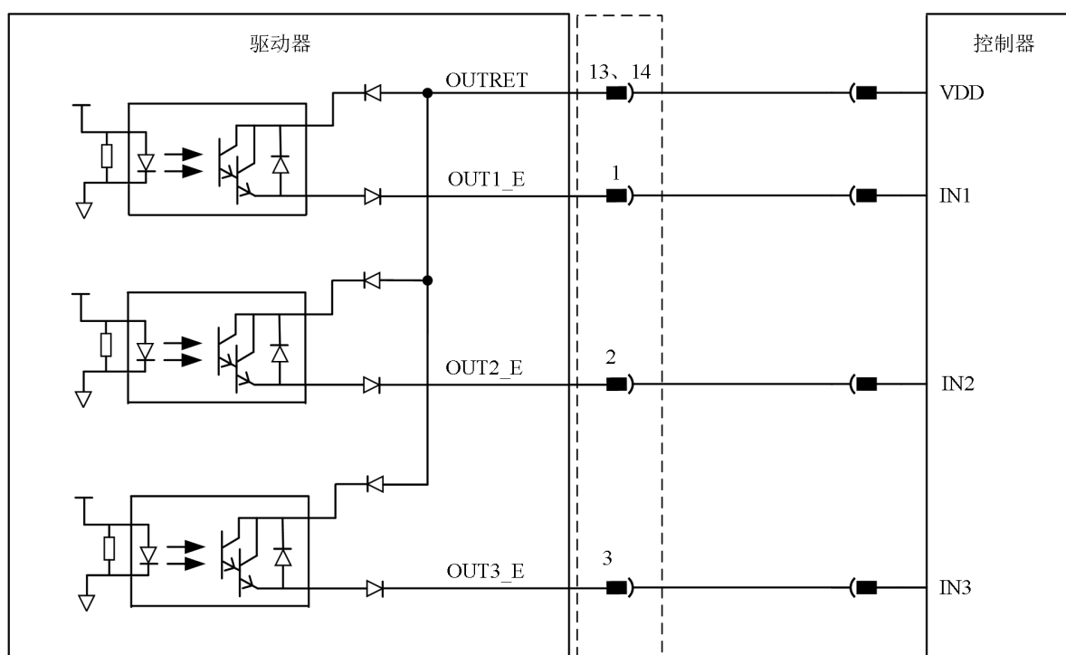
图 4-40 源型输出接线图
