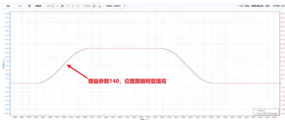
位置环增益 140
