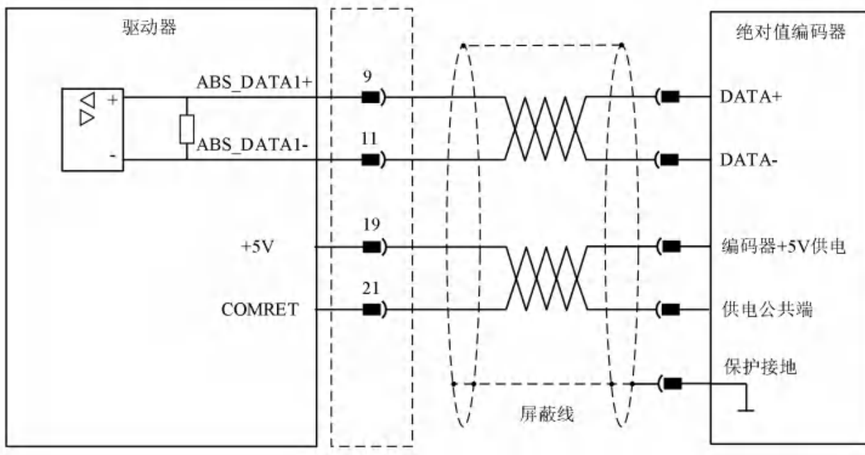
图 4-23 不带时钟信号编码器接线示意图
