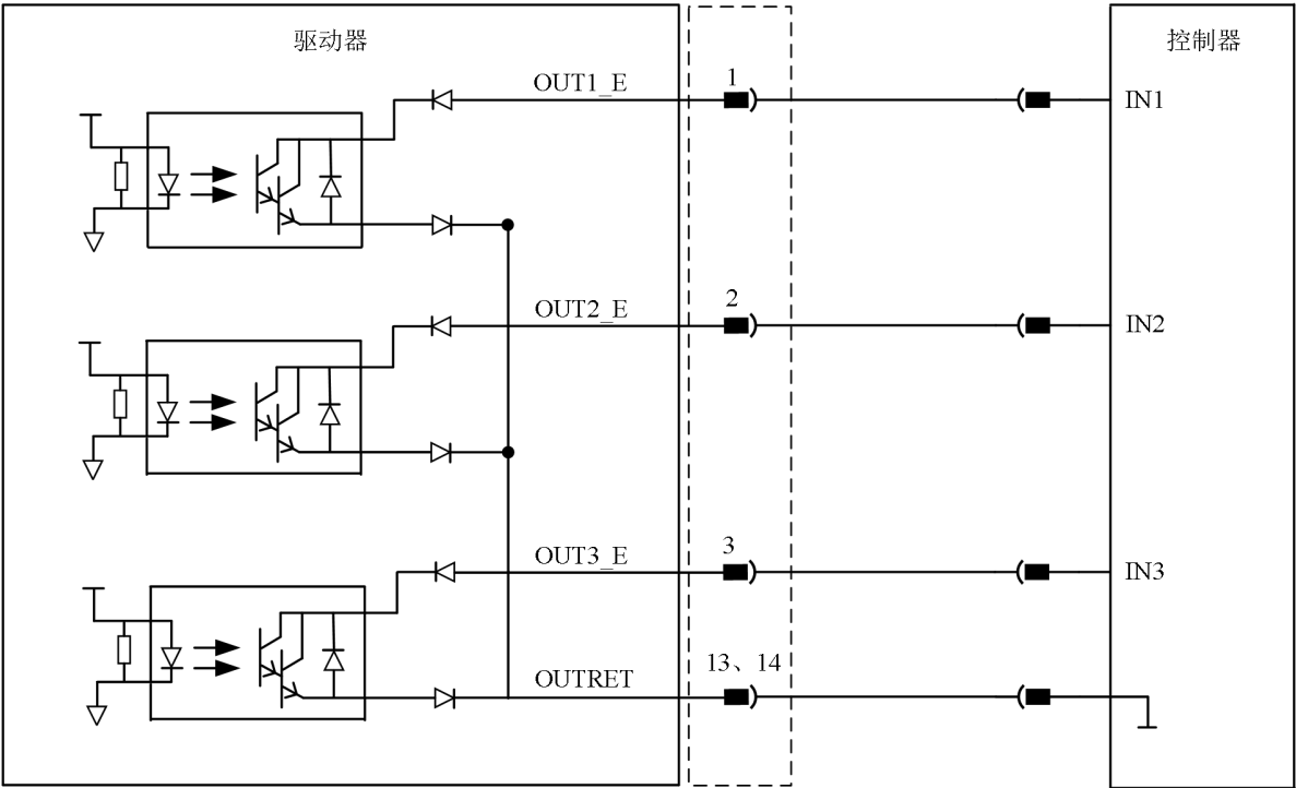
图 4-41 漏型输出接线图
