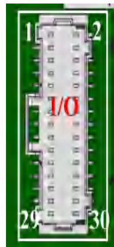
EtherCAT 版 200V 端子脚位示意
