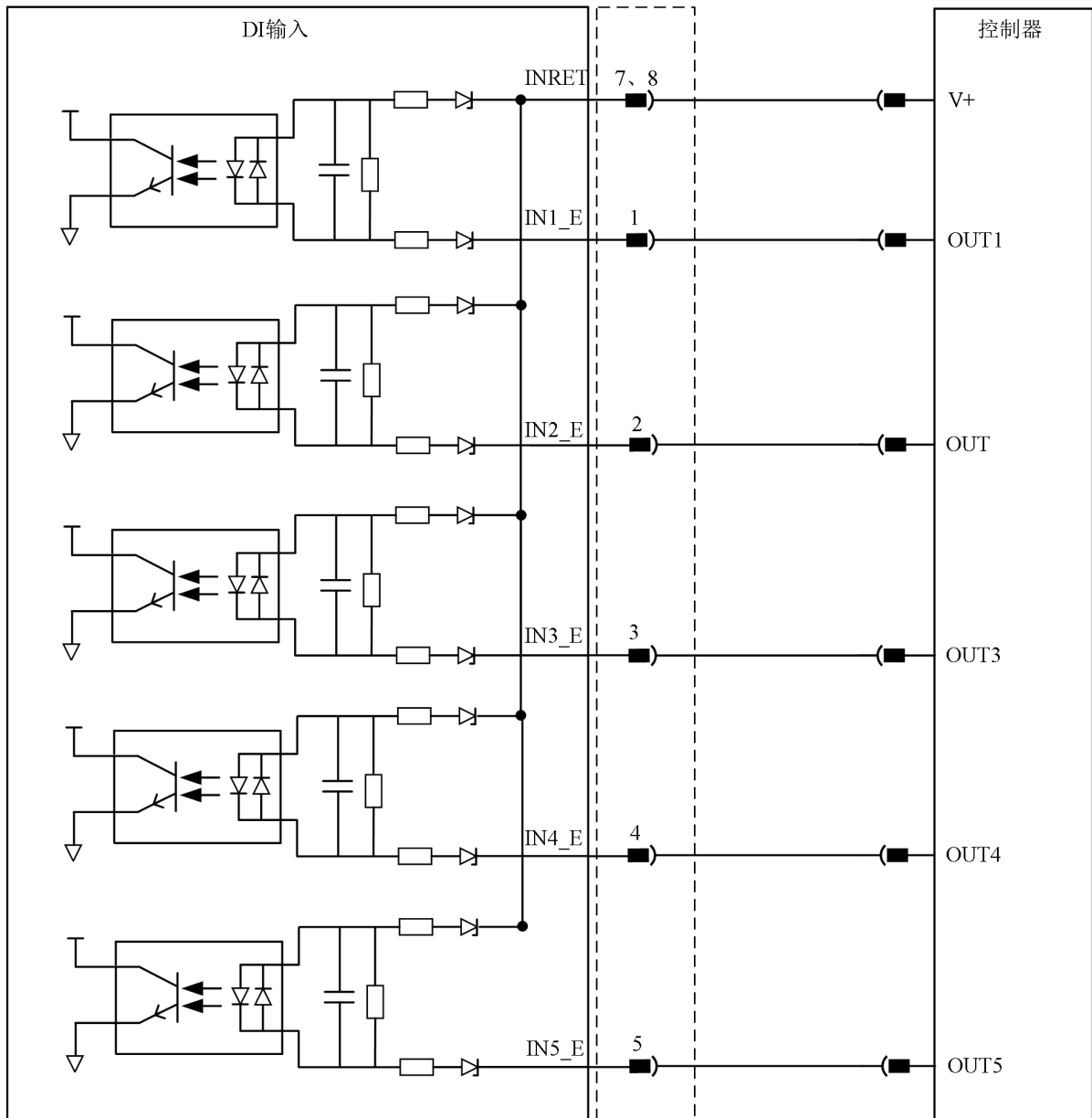
图 4-38 漏型输入接线图
