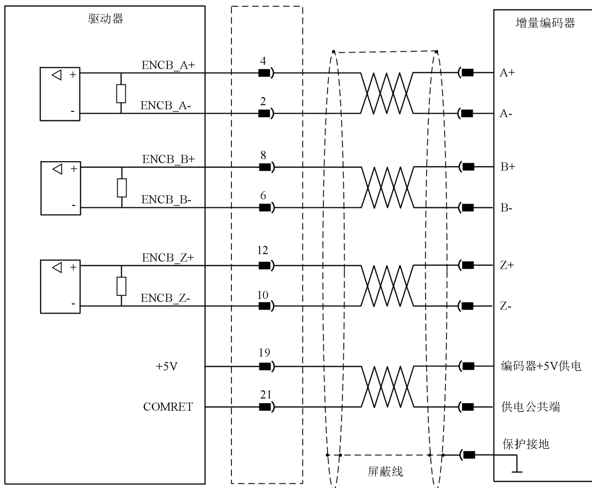
图 4-48 增量编码器接线示意图
