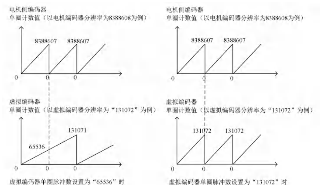
图 1-6 虚拟编码器单圈脉冲数不同配置下计数周期对比示意图
