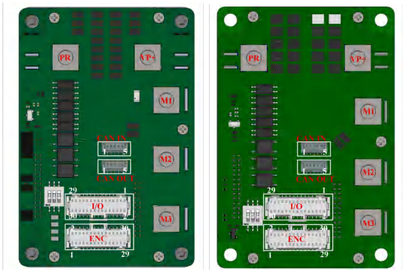
CAN 版 100V 端子脚位示意
