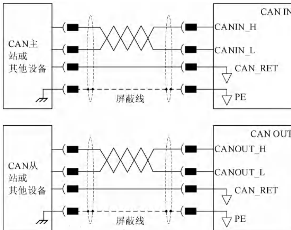
图 4-34 CAN/CAN FD 通讯接线示意图
