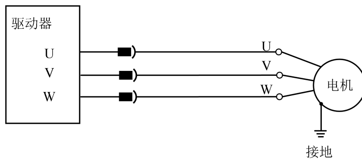
图 4-5 电机接线示意图
