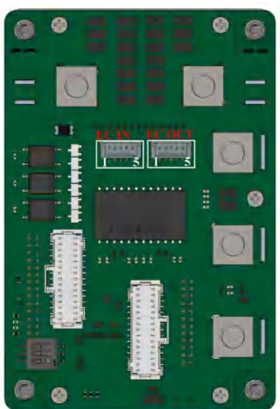
EtherCAT 版 100V 端子脚位示意
