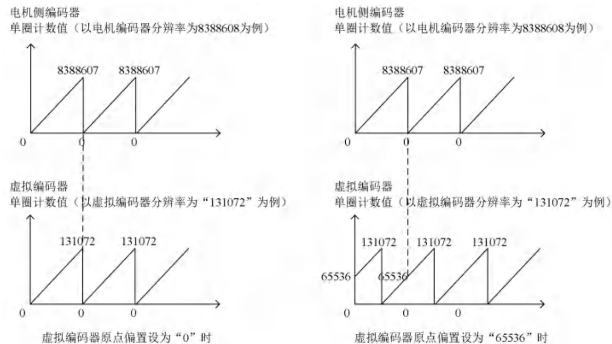
图 1-8 虚拟编码器原点偏置计数对应关系示意图
