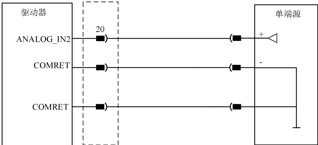
图 4-19 模拟量 2 接线示意图
