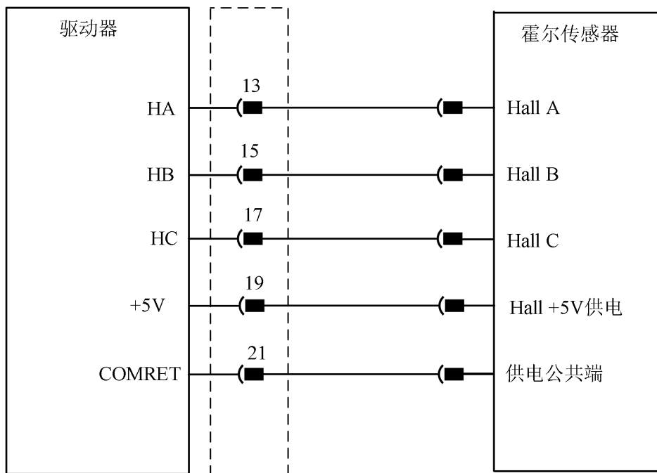
图 4-51 单霍尔接线示意图
