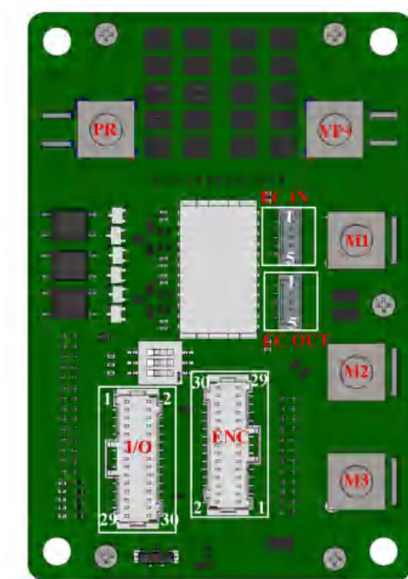
EtherCAT 版 200V 端子脚位示意
