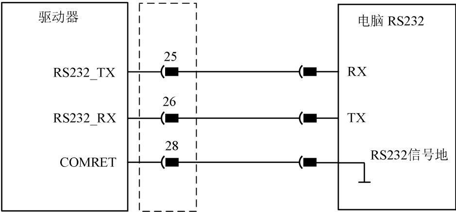
图 4-20 RS232 接线示意图
