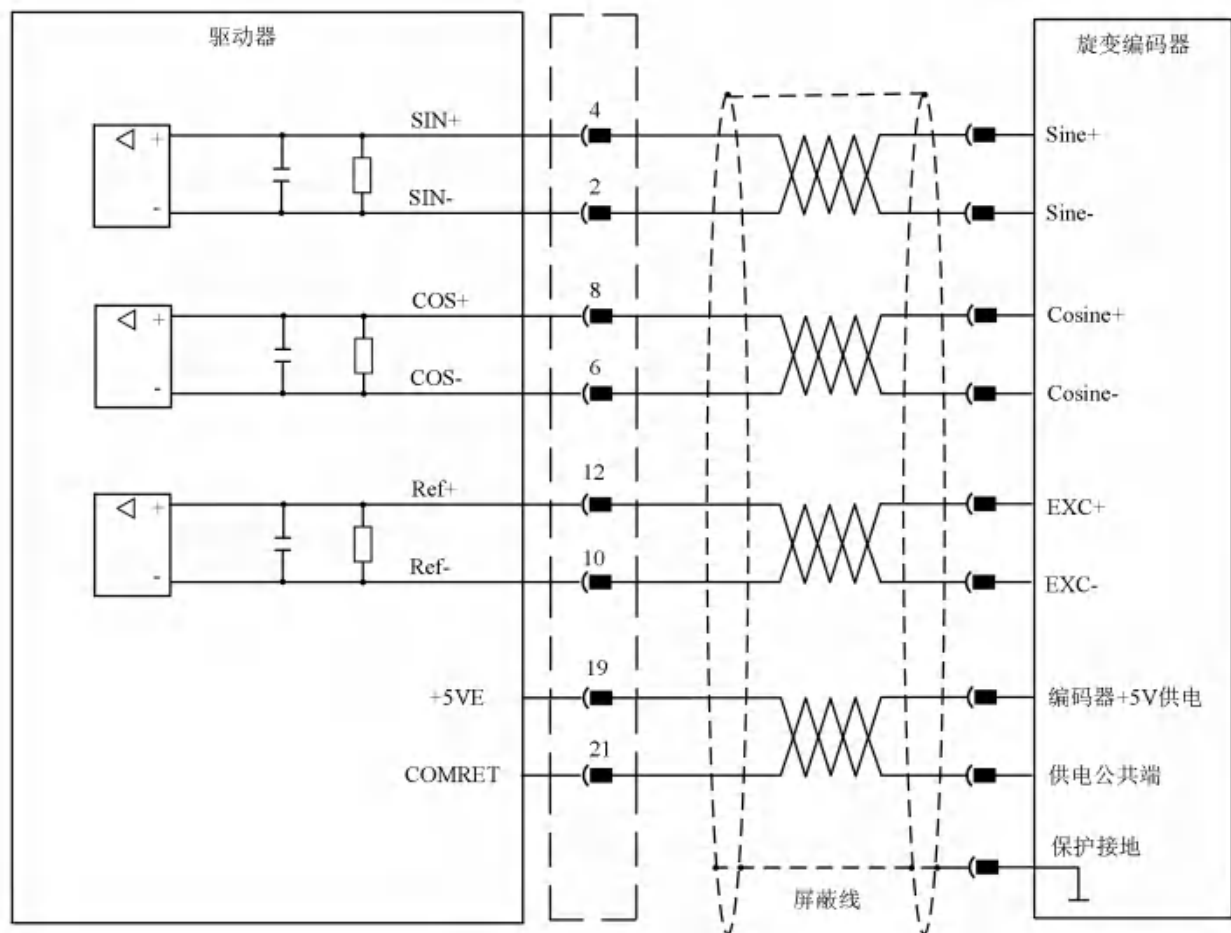
图 4-52 旋变编码器接线示意图
