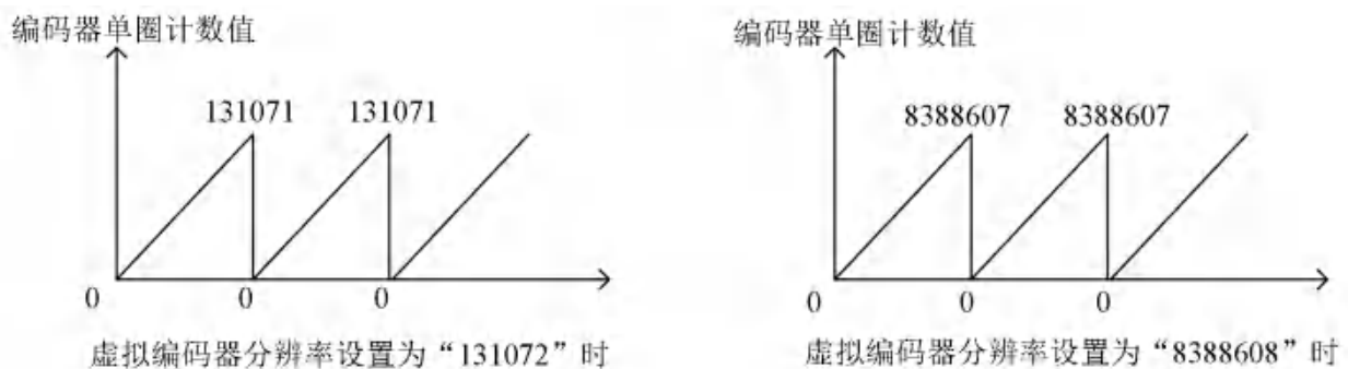
图 1-5 虚拟编码器单圈计数值周期示意图
