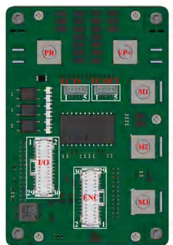
EtherCAT 版 100V 端子脚位示意
