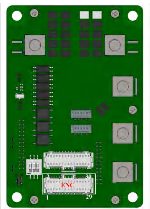
CAN 版 200V 端子脚位示意
