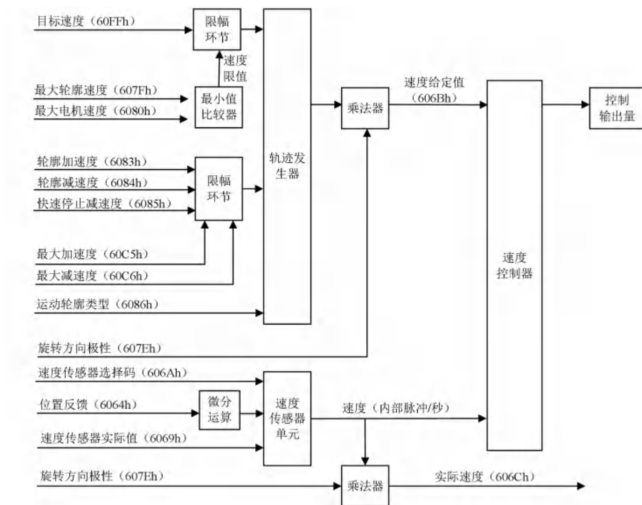
图 9-6 轮廓速度模式 (PV) 控制框图
