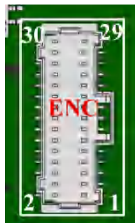
EtherCAT 版 200V 端子脚位示意
