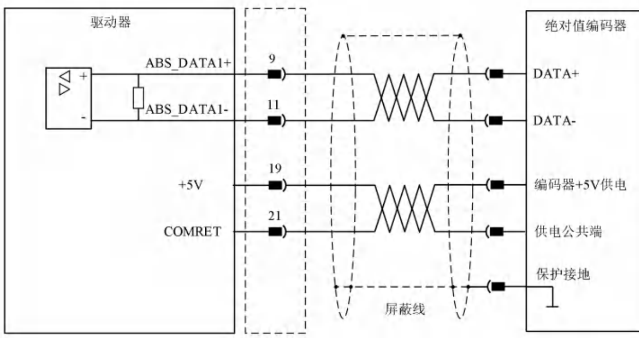
图 4-49 不带时钟信号编码器接线示意图
