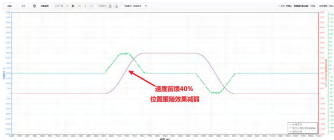
速度前馈 40%
