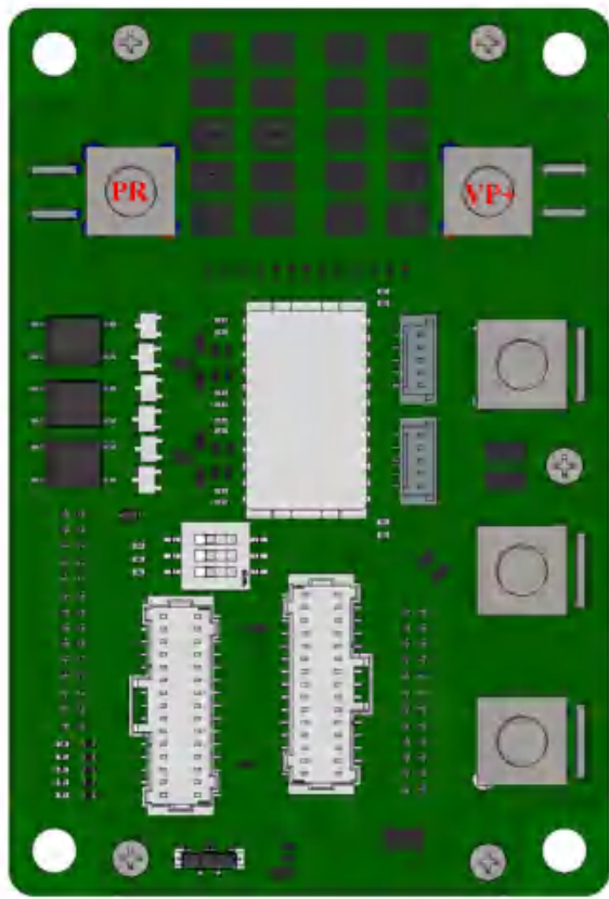
EtherCAT 版 200V 端子脚位示意
