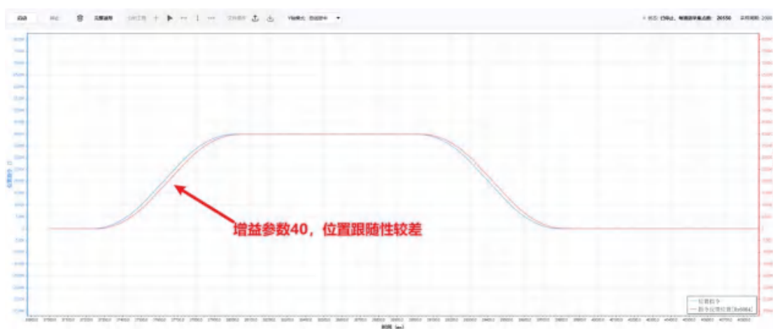
位置环增益 40
