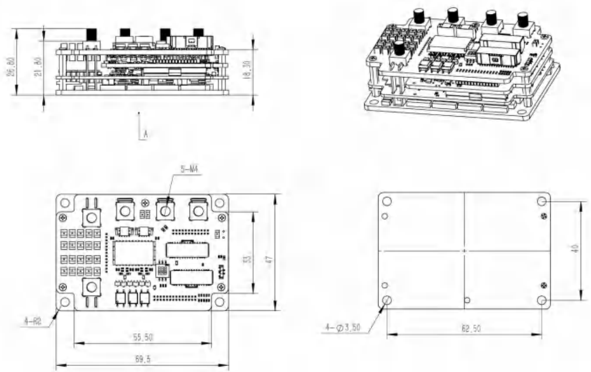
图 1-7 EtherCAT（200V）版本驱动器安装图纸
