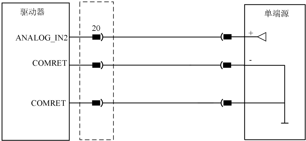
图 4-45 模拟量 2 接线示意图
