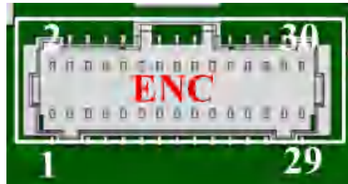
CAN 版 200V 端子脚位示意
