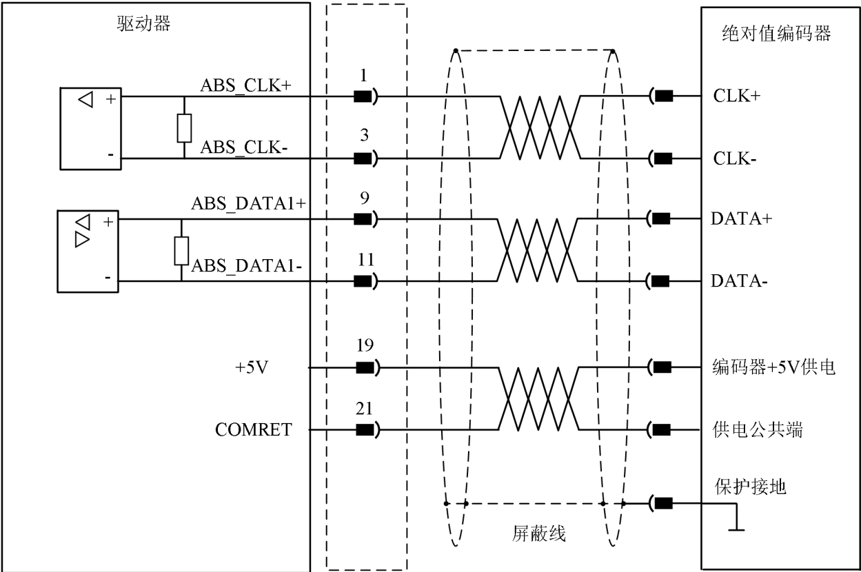
图 4-50 带时钟信号编码器接线示意图
