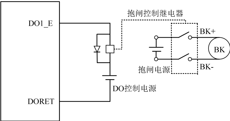
图 4-17 抱闸接线图
