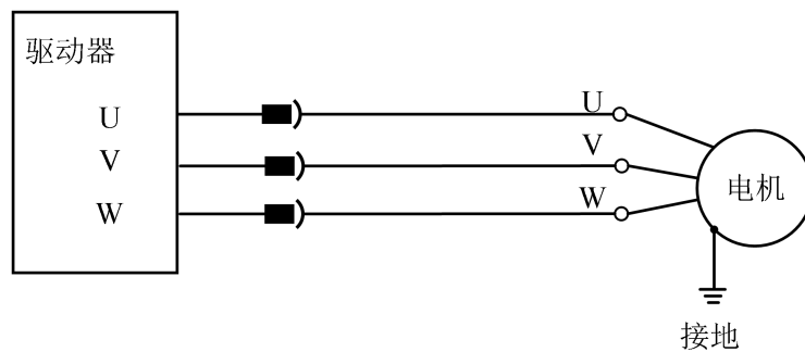
图 4-31 电机接线示意图
