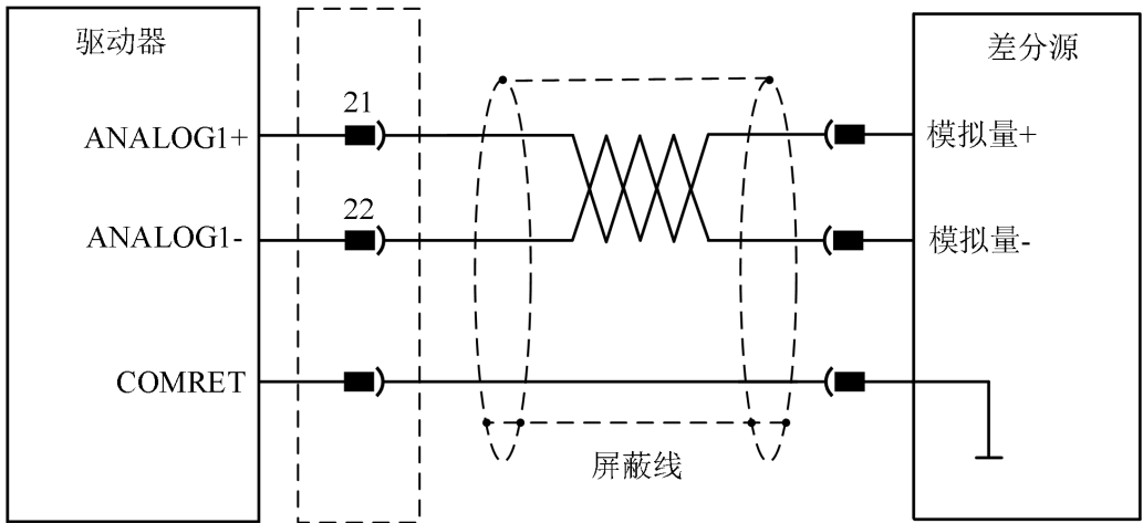
图 4-44 模拟量 1 接线示意图
