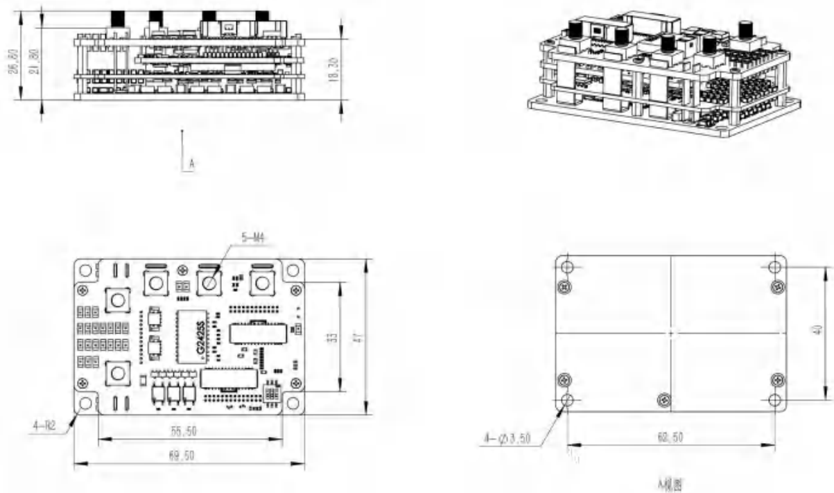
图 1-6 EtherCAT（100V）版本驱动器安装图纸
