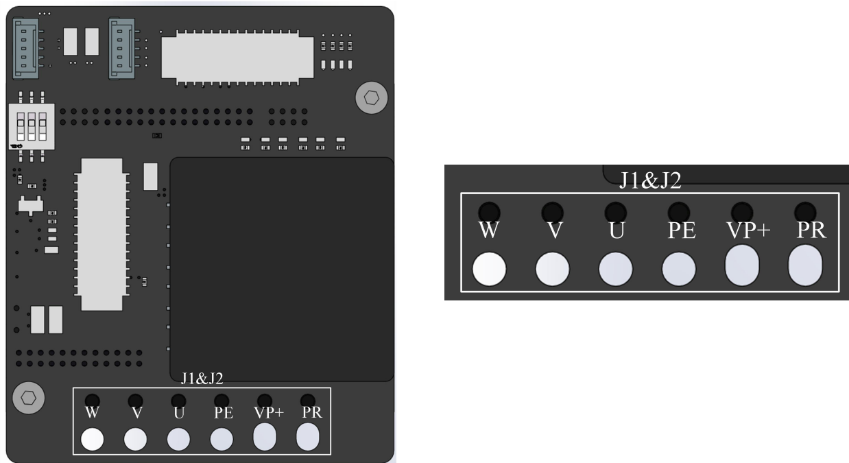
图 4-2 电源接口示意图
