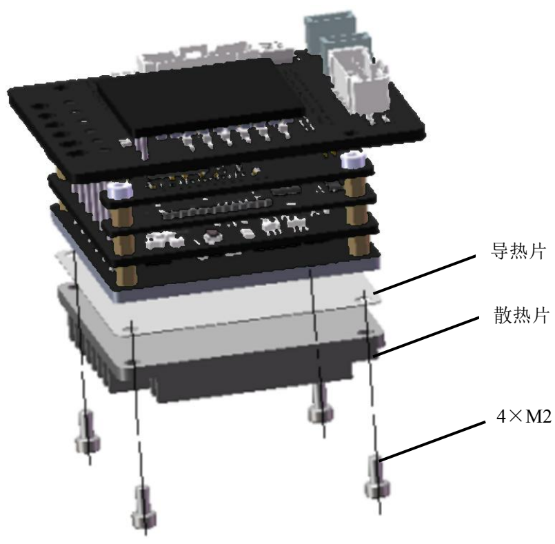
图 3-1 散热附件安装示意图
