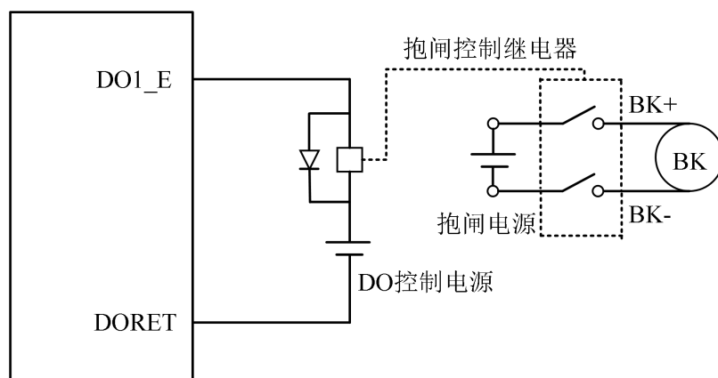
图 8-12 抱闸接线图
