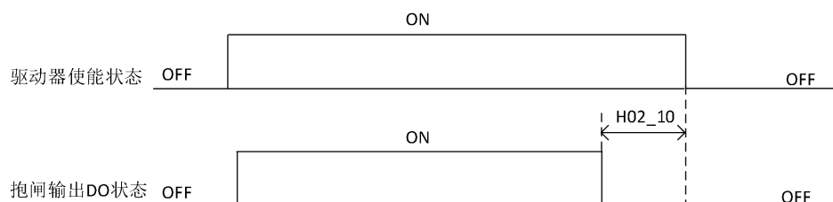
图 8-13 抱闸输出时序图
