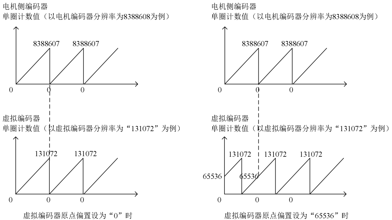
图 1-4 虚拟编码器原点偏置计数对应关系示意图
