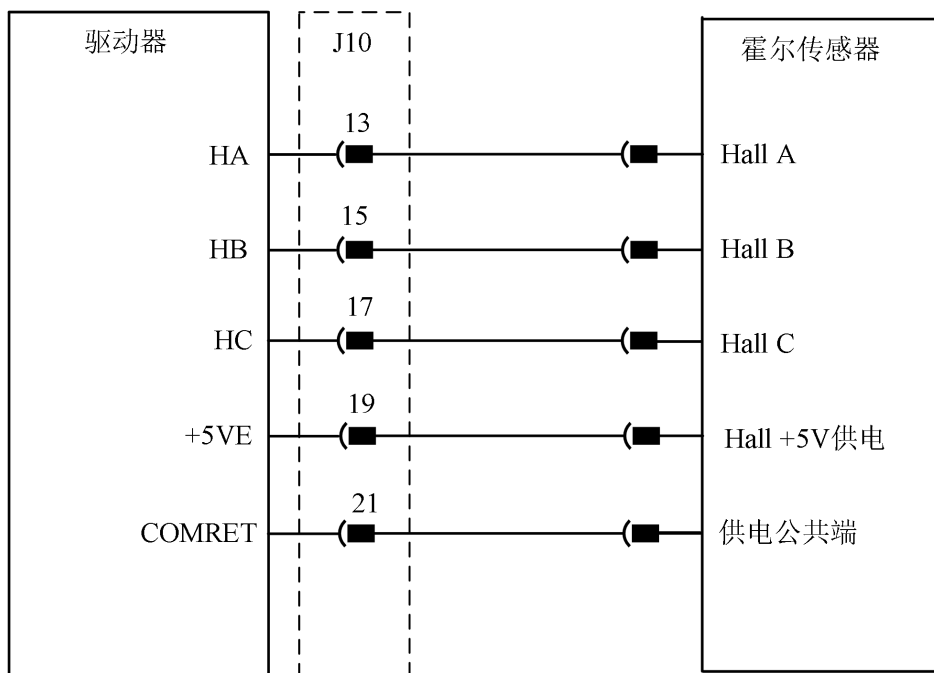
图 4-25 单霍尔接线示意图
