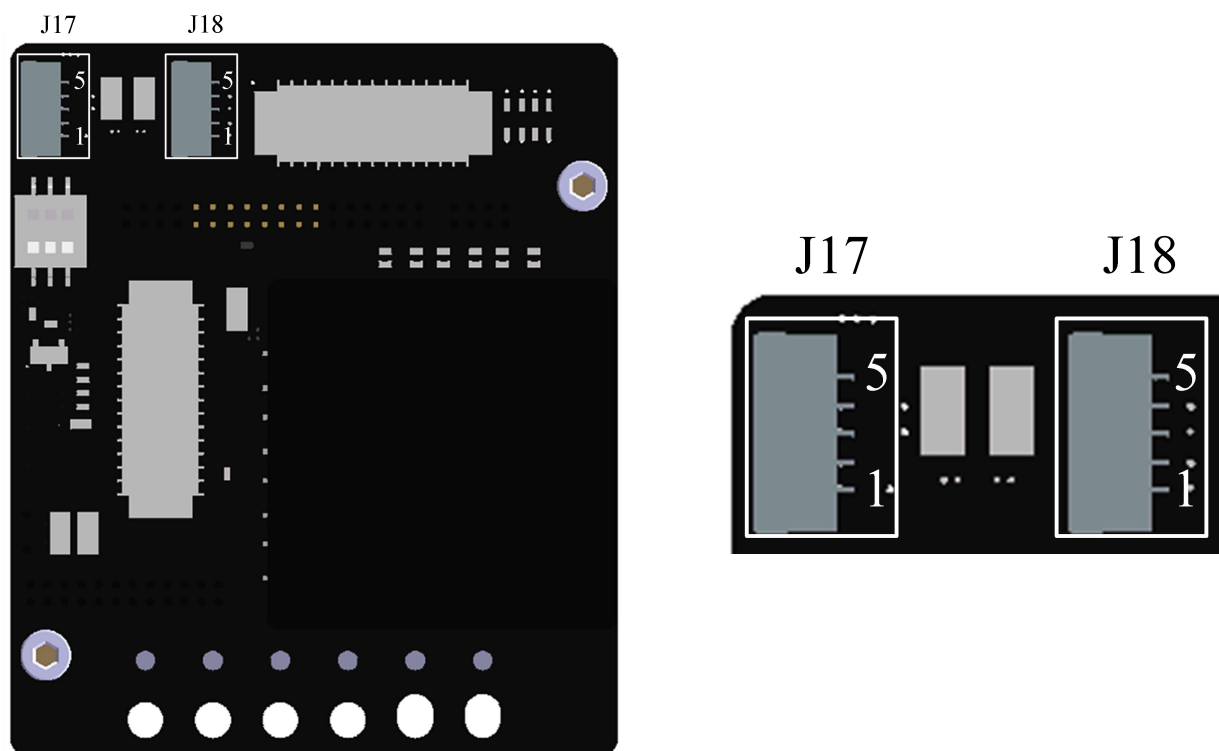
图 4-9 EtherCAT 通讯接口示意图
