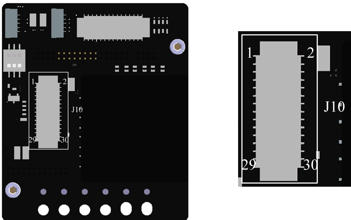
图 4-21 编码器接口定义图
