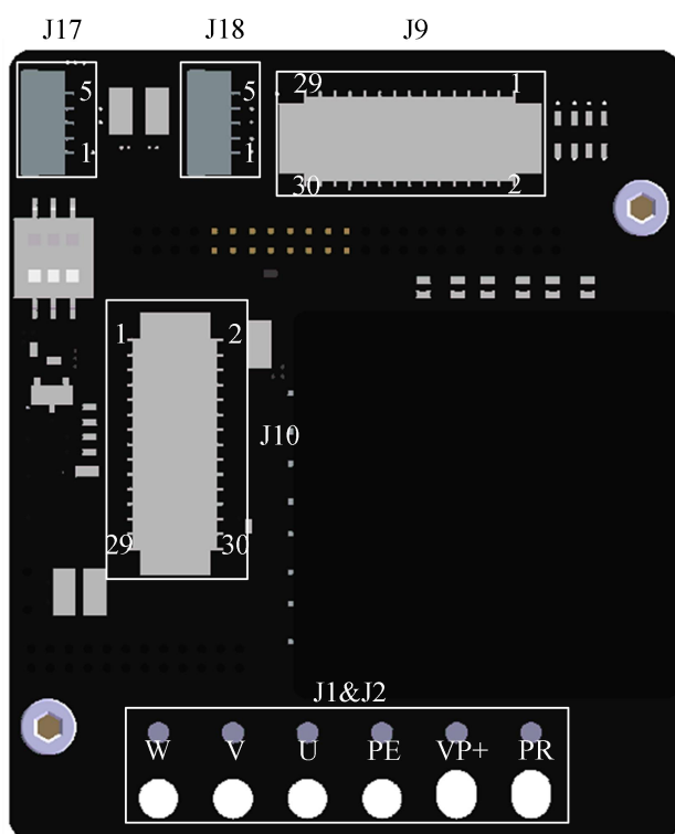
EtherCAT 端子脚位示意图
