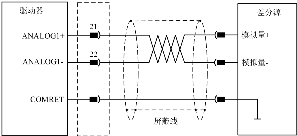
图 4-17 模拟量 1 接线示意图
