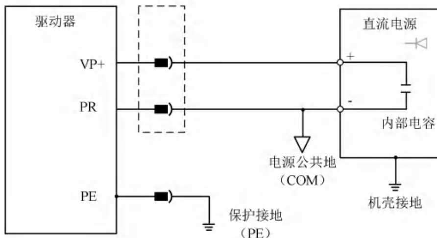
图 4-4 单电源供电接线示意图
