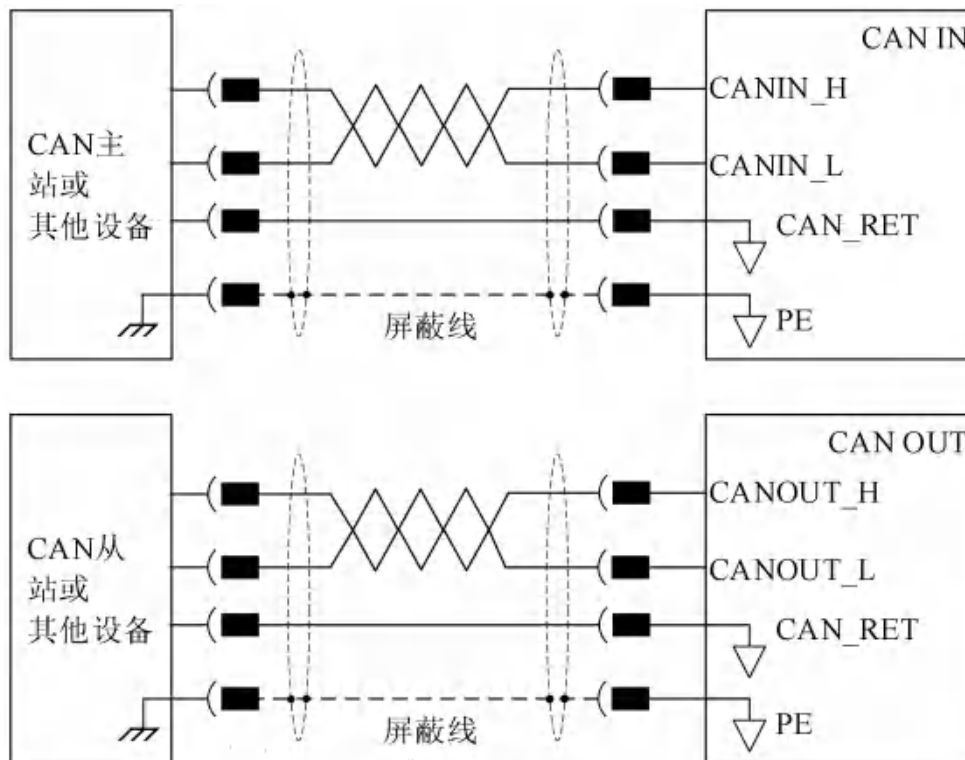
图 4-33 CAN/CAN FD 通讯接线示意图
