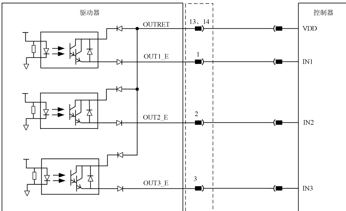
图 4-37 源型输出接线图
