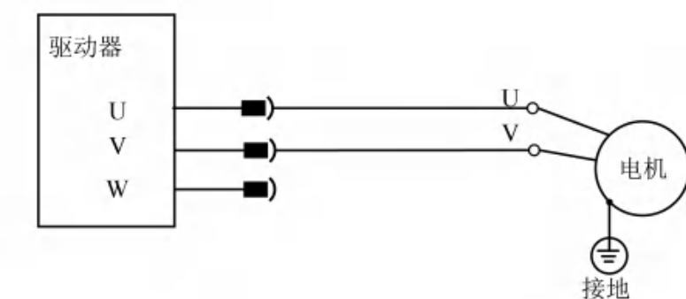
图 4-7 电机接线示意图
