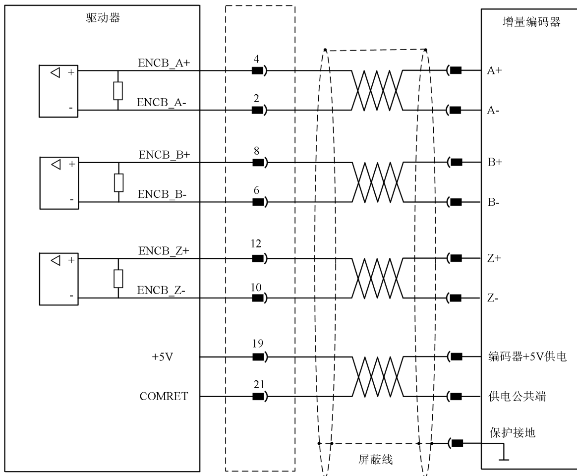
图 4-21 增量编码器接线示意图
