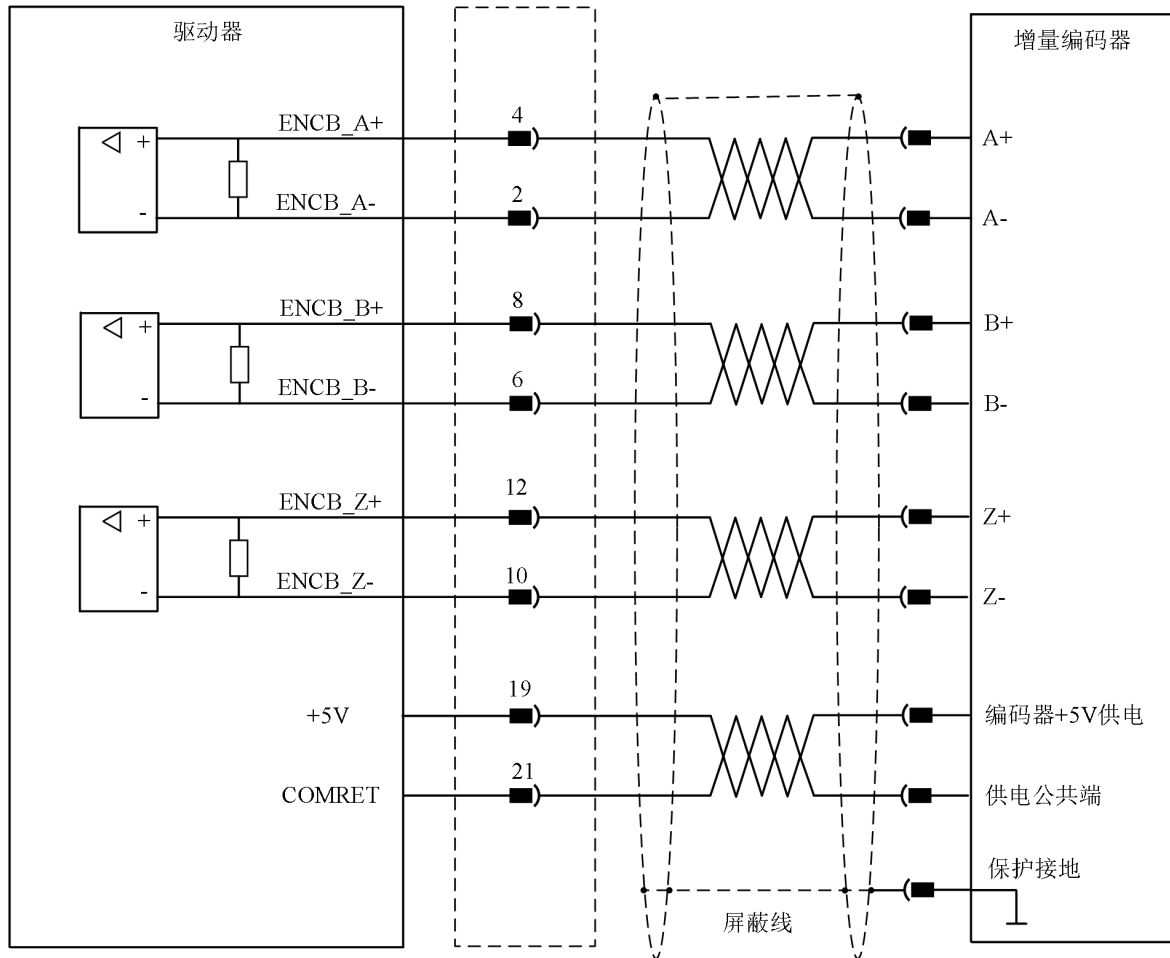
图 4-45 增量编码器接线示意图
