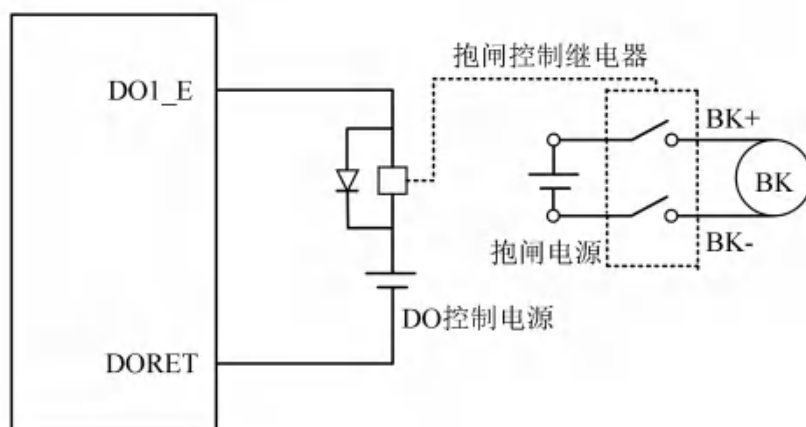
图 8-17 抱闸接线图
