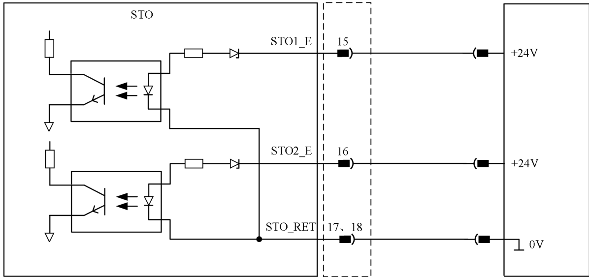
图 4-15 STO 接线示意图
