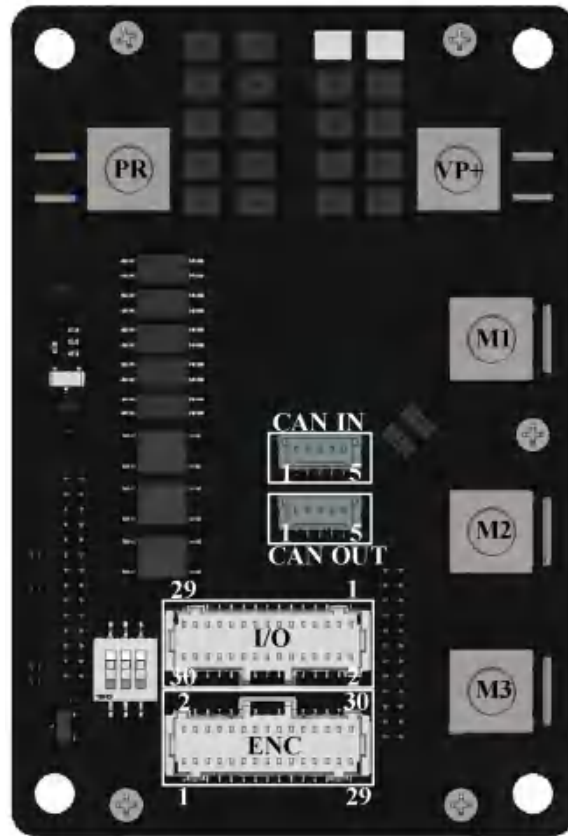
CAN 版 200V 端子脚位示意
