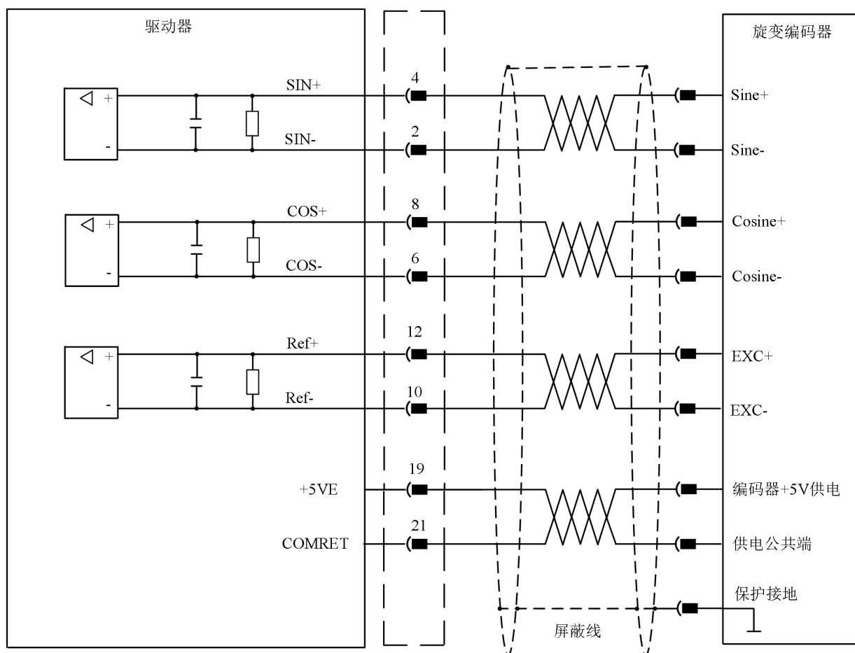
图 4-25 旋变编码器接线示意图
