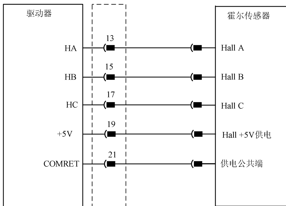
图 4-24 单霍尔接线示意图
