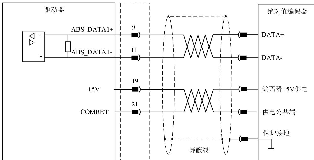
图 4-46 不带时钟信号编码器接线示意图
