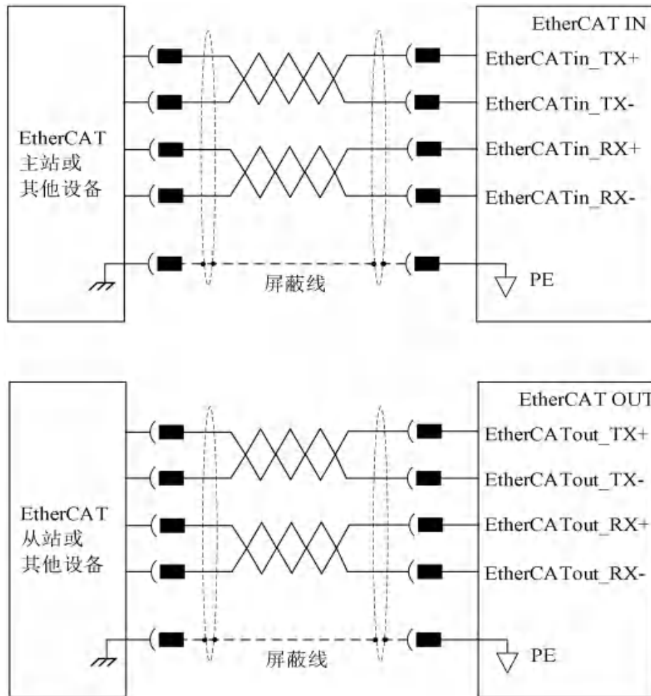
图 4-9 EtherCAT 通讯接线示意图
