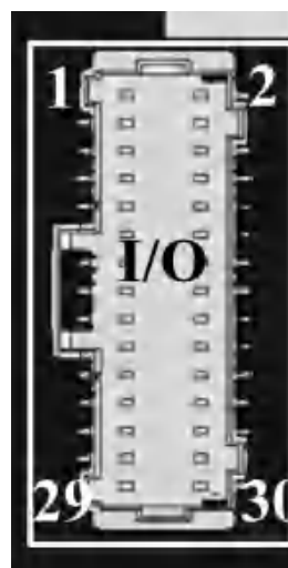
EtherCAT 版 200V 端子脚位示意
