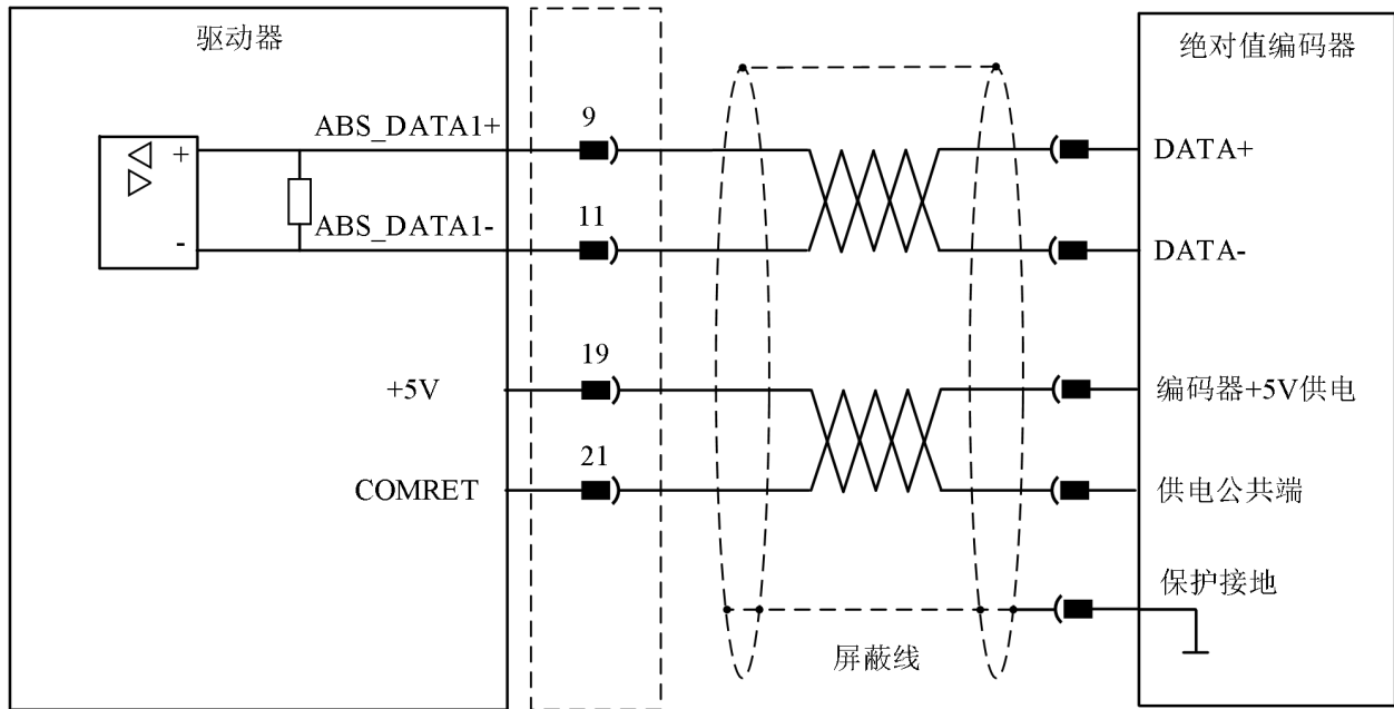
图 4-22 不带时钟信号编码器接线示意图
