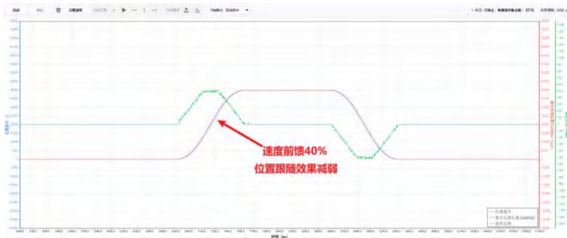
速度前馈 40%
