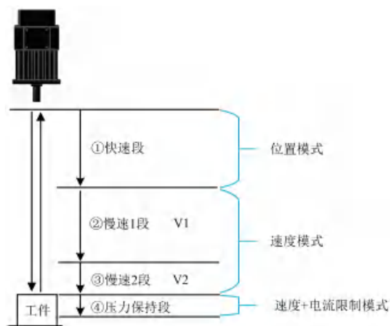
图 8-2 力控运行阶段示意图
