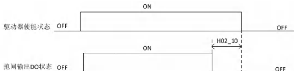
图 8-18 抱闸输出时序图
