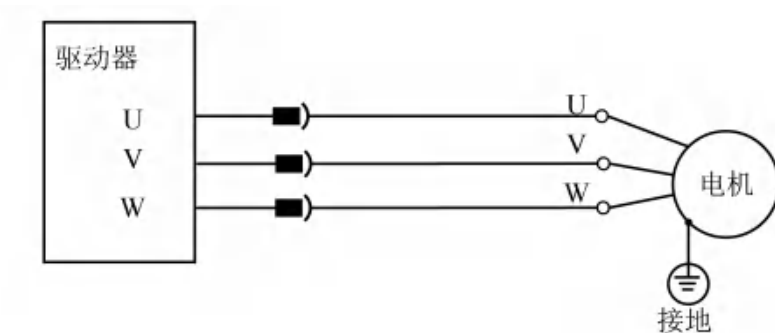
图 4-6 电机接线示意图
