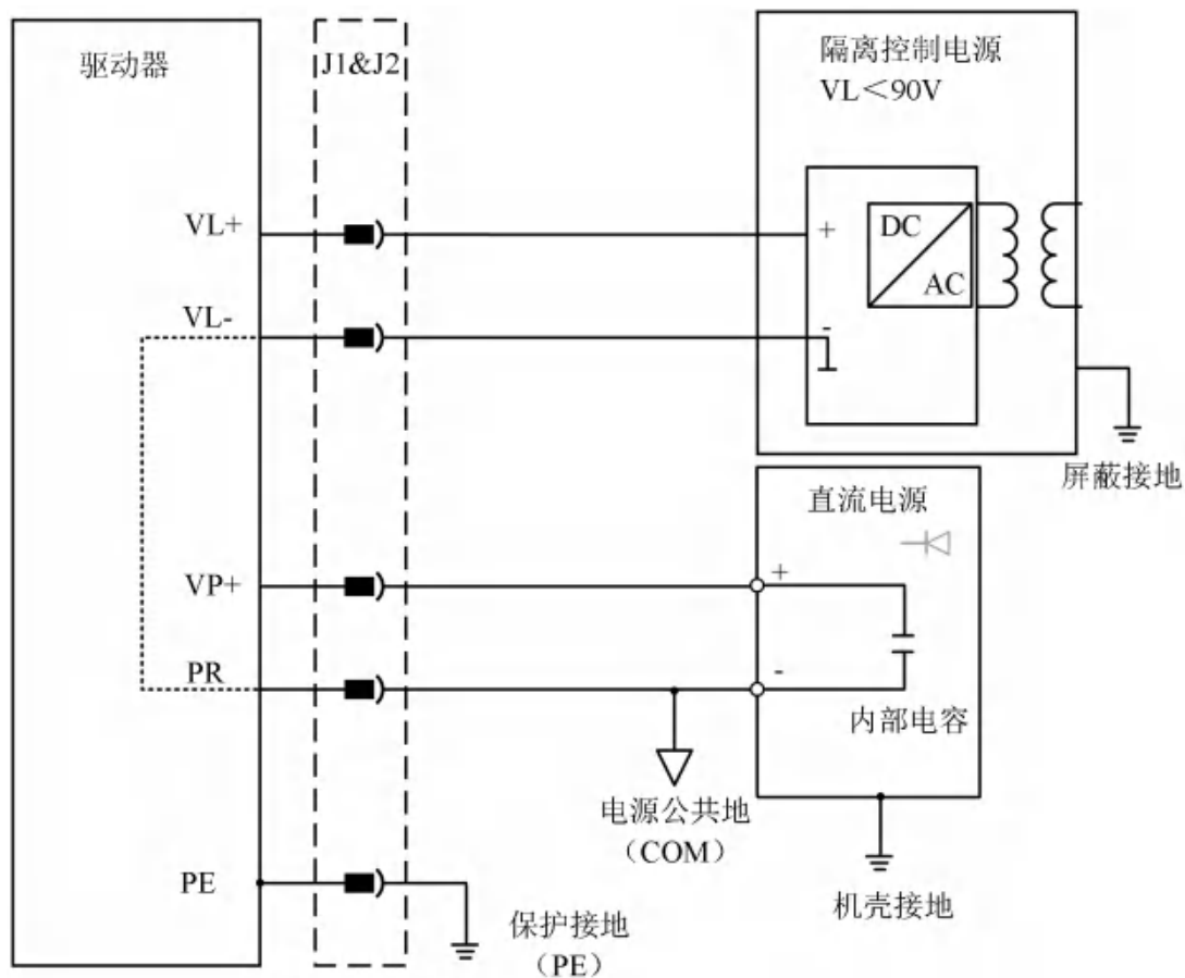
图 4-3 双电源供电接线示意图
