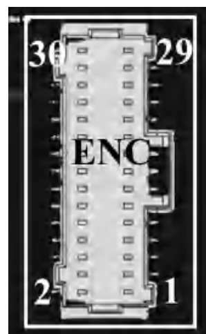
EtherCAT 版 200V 端子脚位示意
