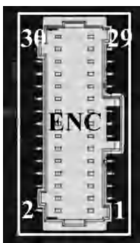
EtherCAT 版 100V 端子脚位示意
