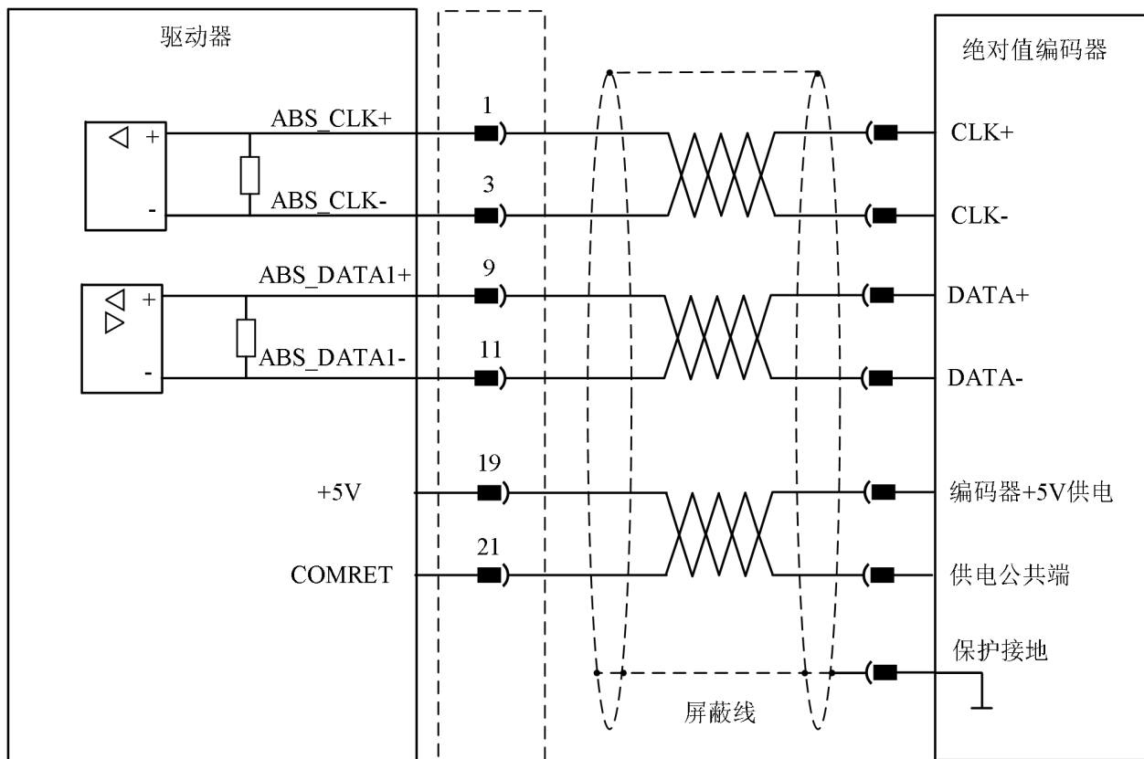
图 4-23 带时钟信号编码器接线示意图
