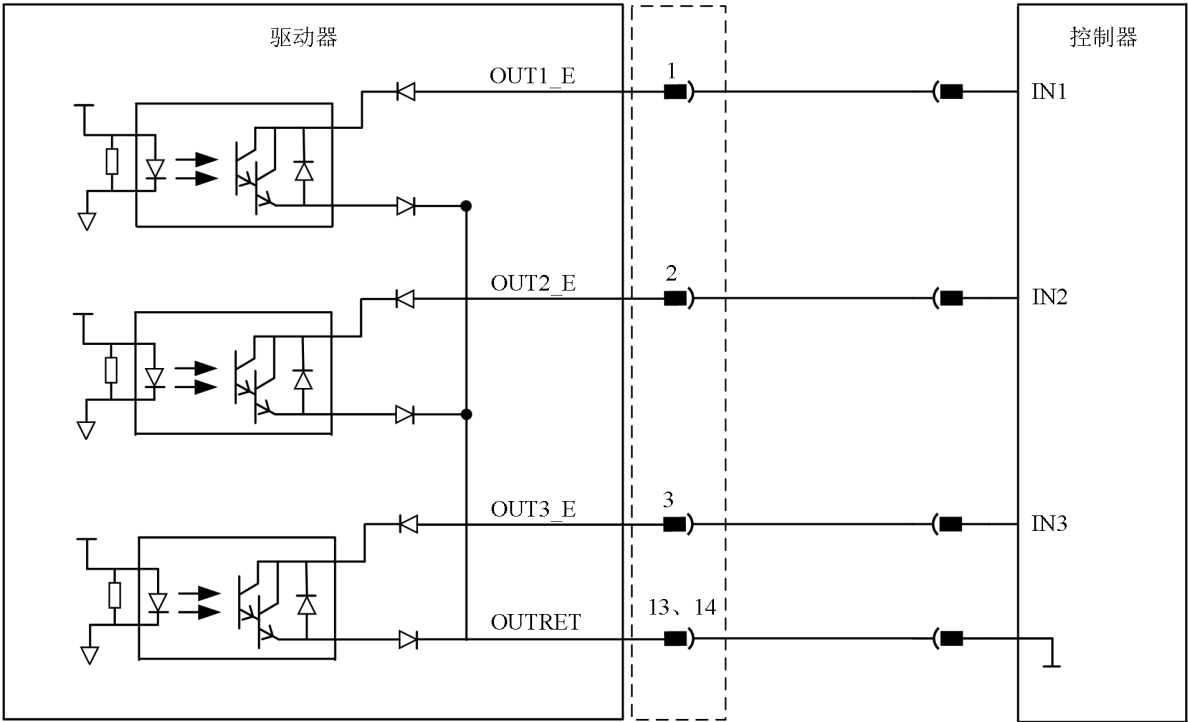
图 4-14 漏型输出接线图
