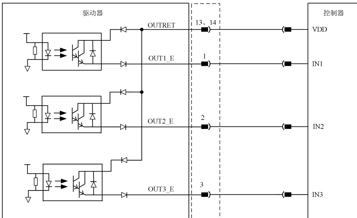
图 4-13 源型输出接线图
