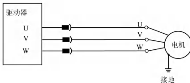
图 4-30 电机接线示意图
