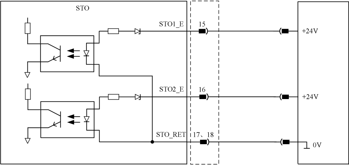
图 4-39 STO 接线示意图
