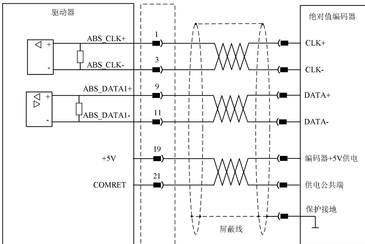
图 4-47 带时钟信号编码器接线示意图
