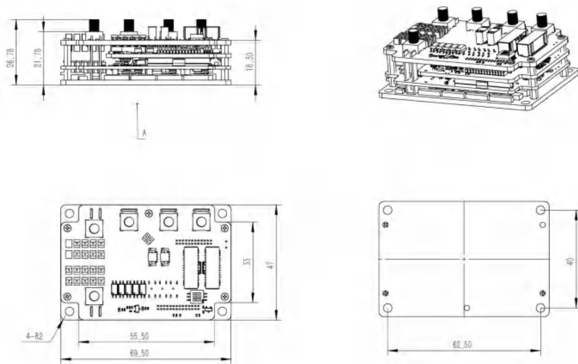
图 1-4 CANopen（200V）版本驱动器安装图纸
