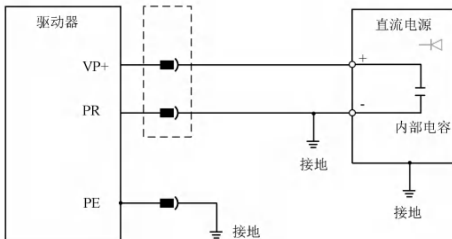
图 4-28 供电接线示意图
