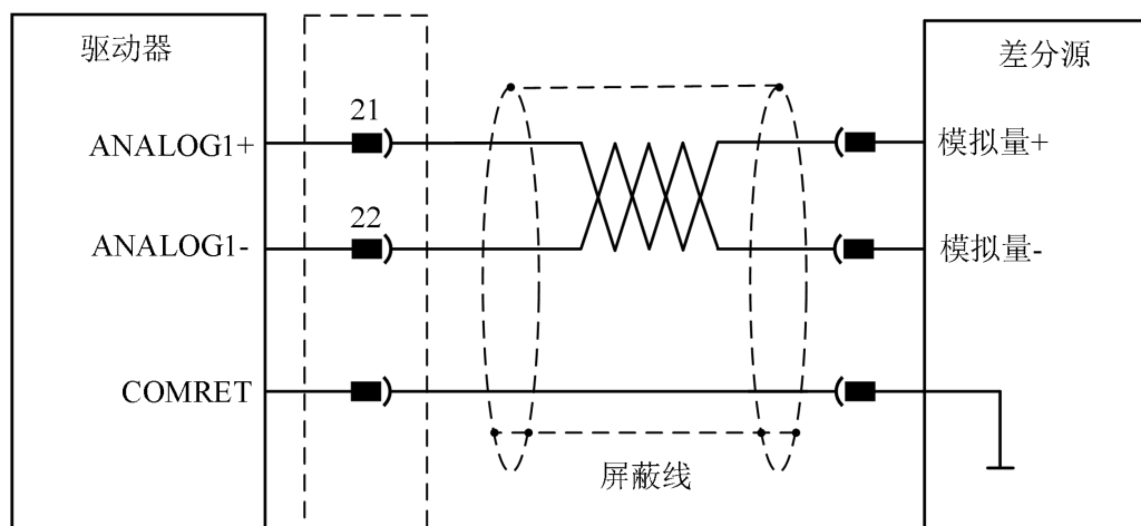
图 4-41 模拟量 1 接线示意图
