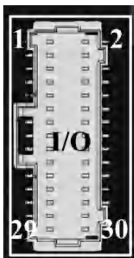
EtherCAT 版 100V 端子脚位示意
