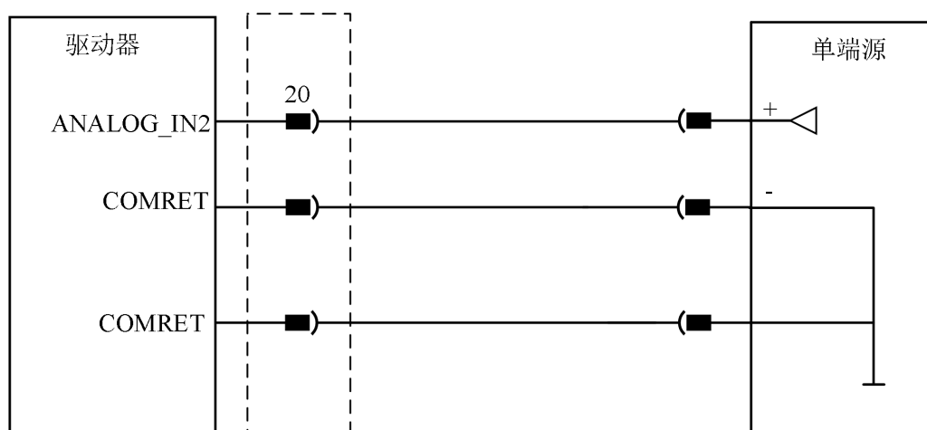
图 4-42 模拟量 2 接线示意图
