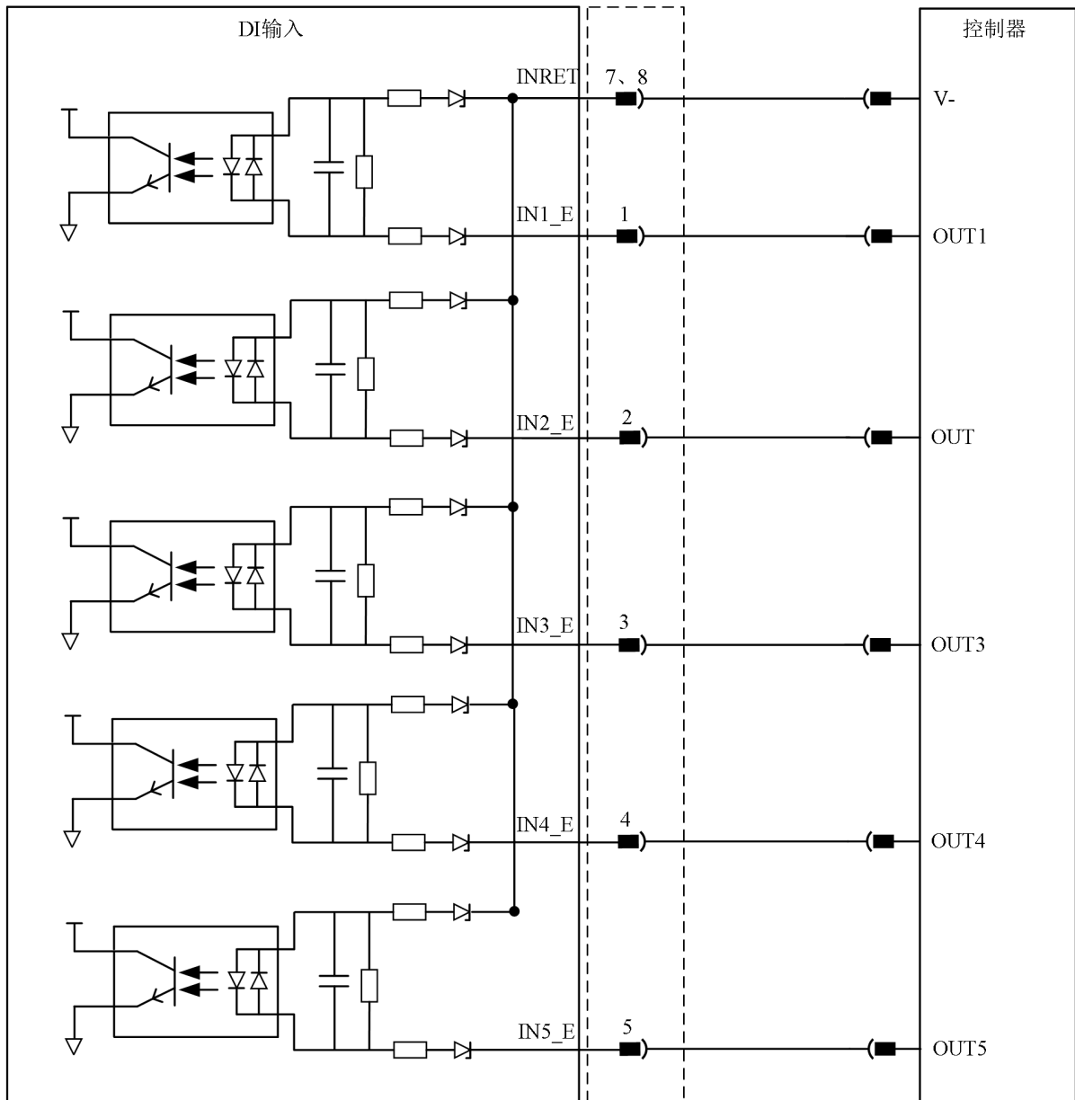
图 4-12 源型输入接线图
