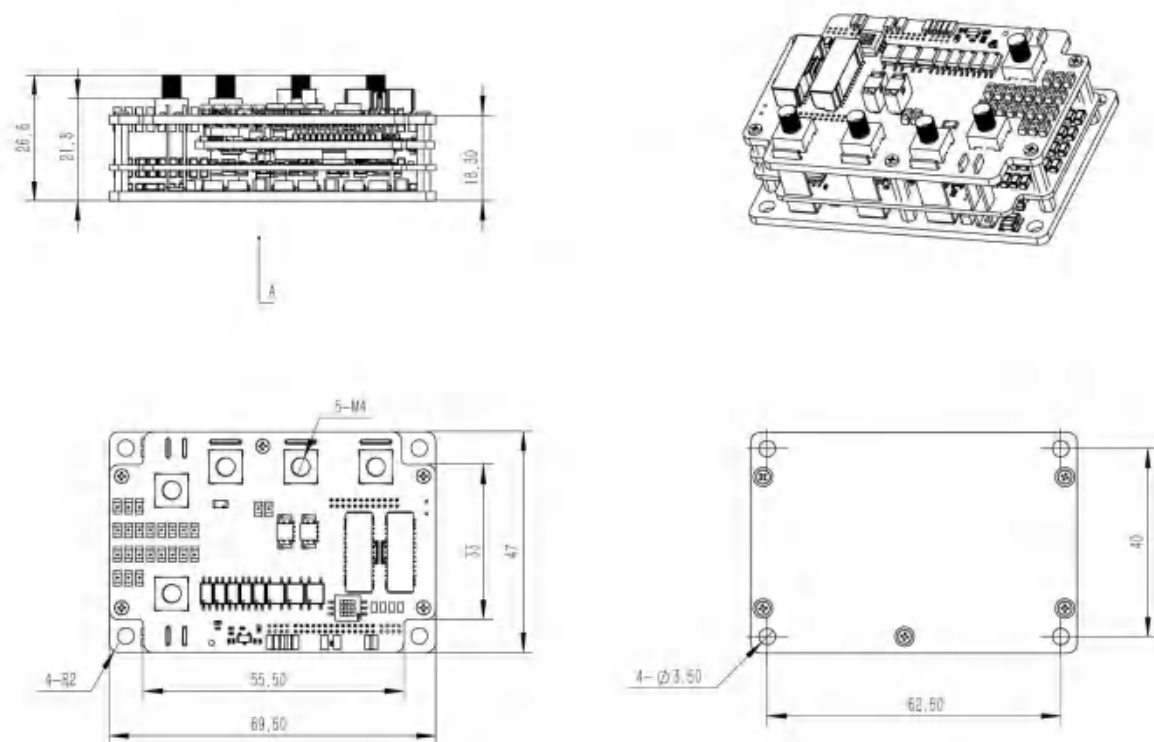
图 1-3 CANopen（100V）版本驱动器安装图纸
