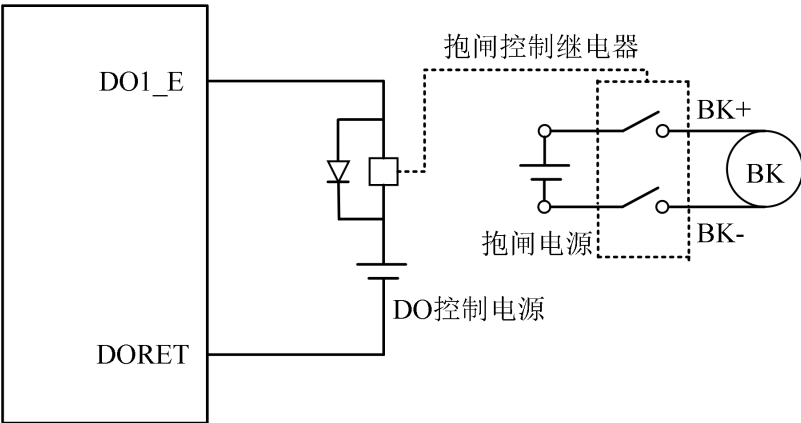
图 4-40 抱闸接线图
