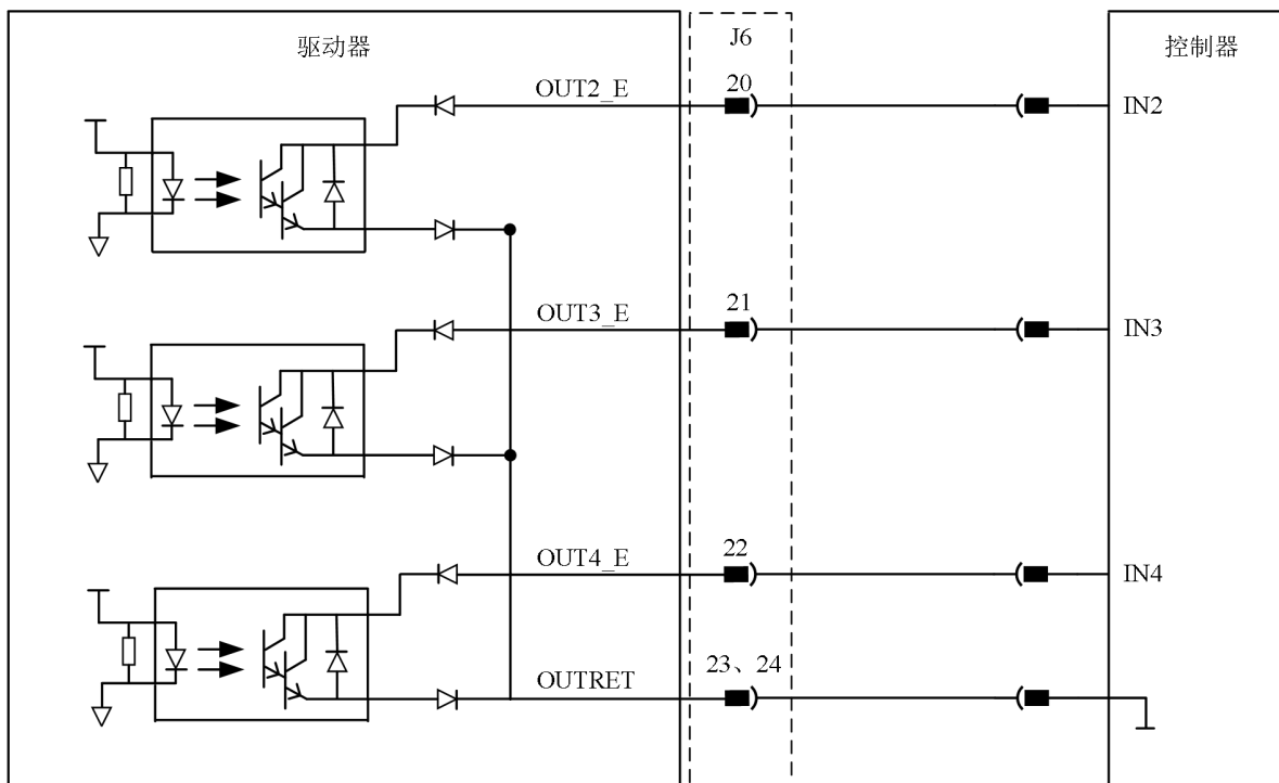
图 4-17 漏型输出接线图
