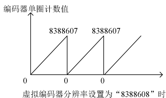
图 1-5 虚拟编码器单圈计数值周期示意图
