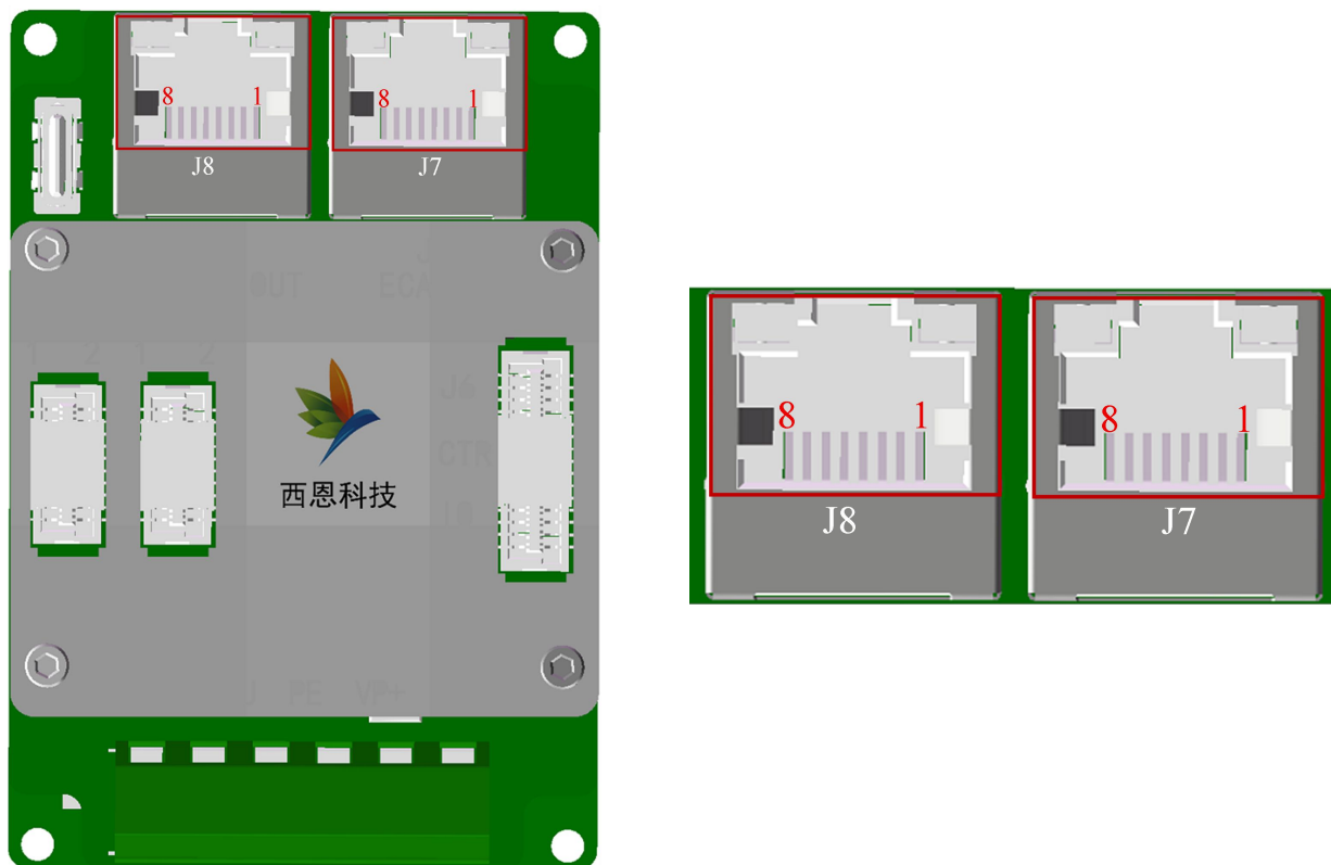
图 4-7 CAN/CAN FD 通讯接口示意图
