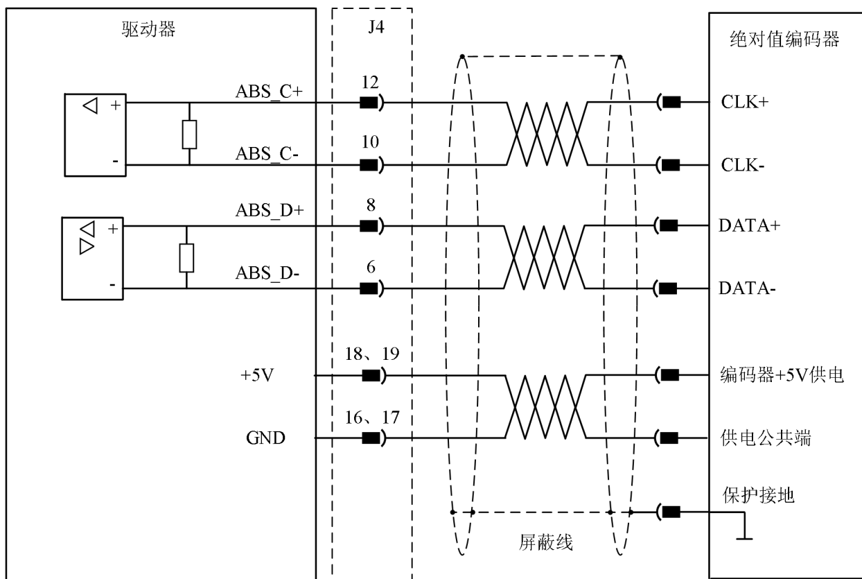
图 4-27 带时钟信号 BiSS-C/SSI 编码器接线示意图
