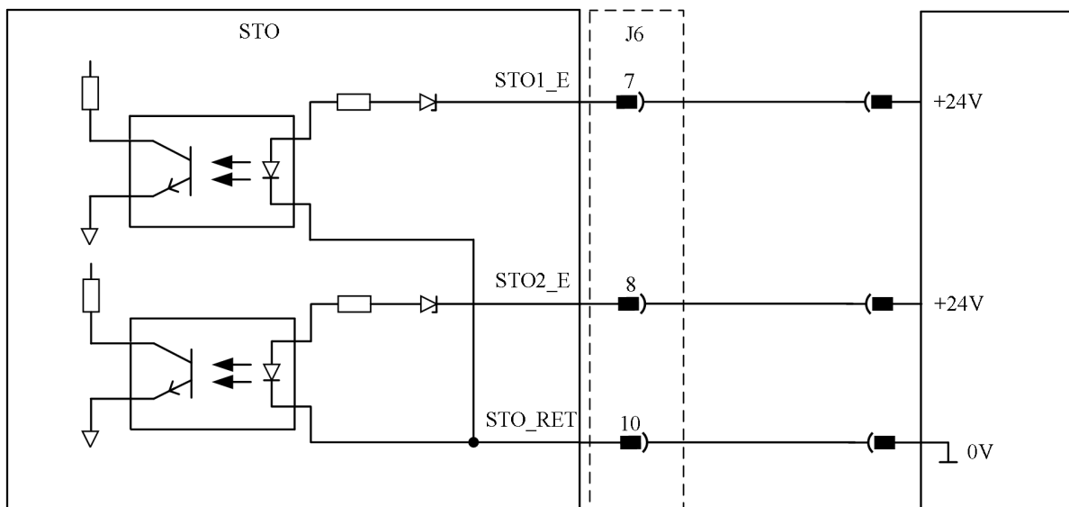
图 4-18 STO 接线示意图
