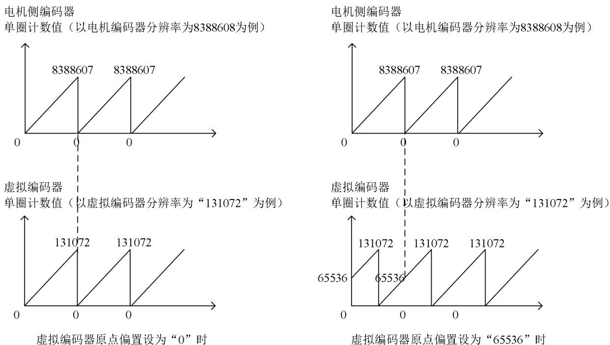
图 1-8 虚拟编码器原点偏置计数对应关系示意图
