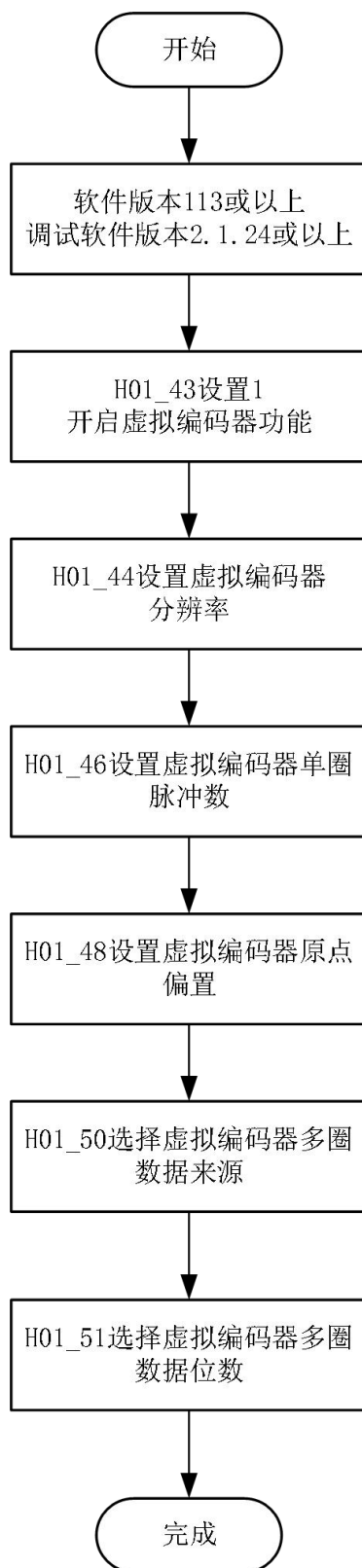
图 1-9 虚拟编码器功能操作流程示意图
