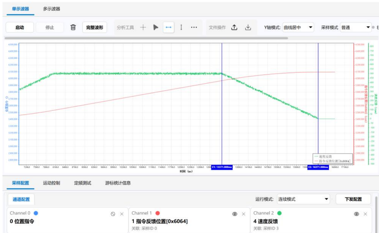
图 1-13 上位机调试软件减速停止波形图
