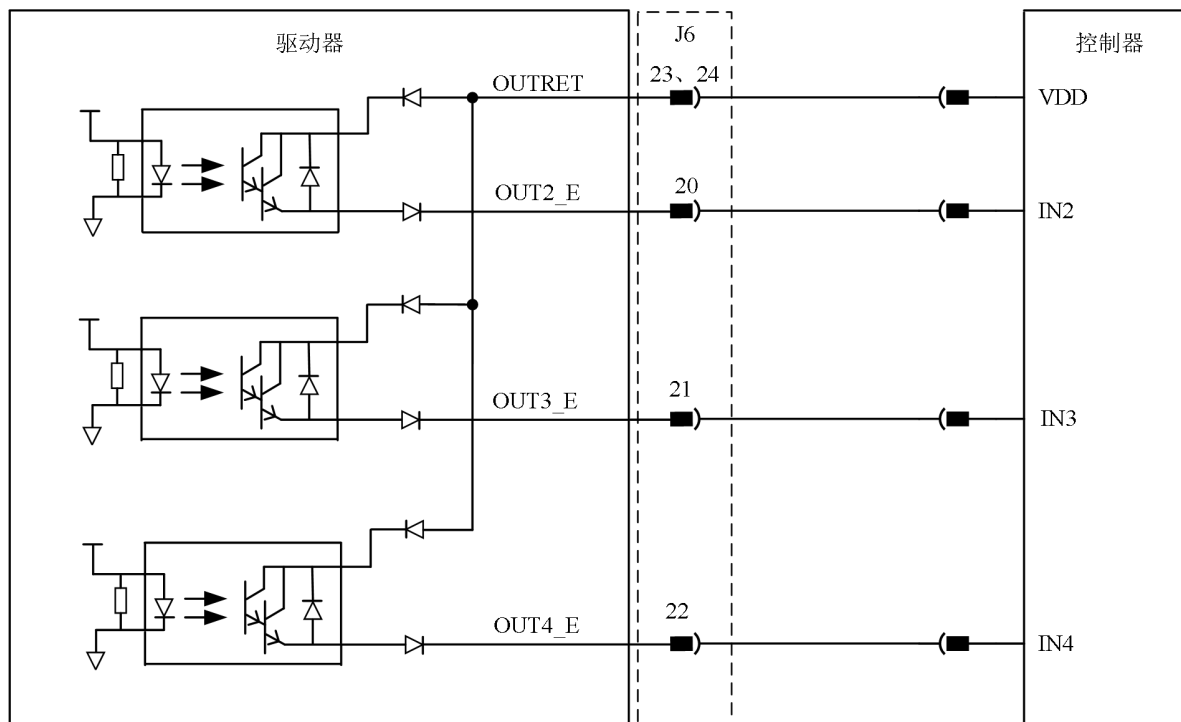
图 4-16 源型输出接线图
