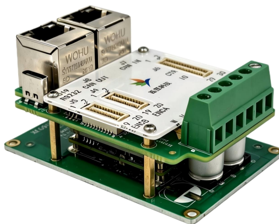
图 1-1 立式端子驱动器外观图
