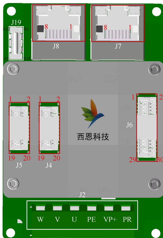
图 4-1 端子脚位示意图
