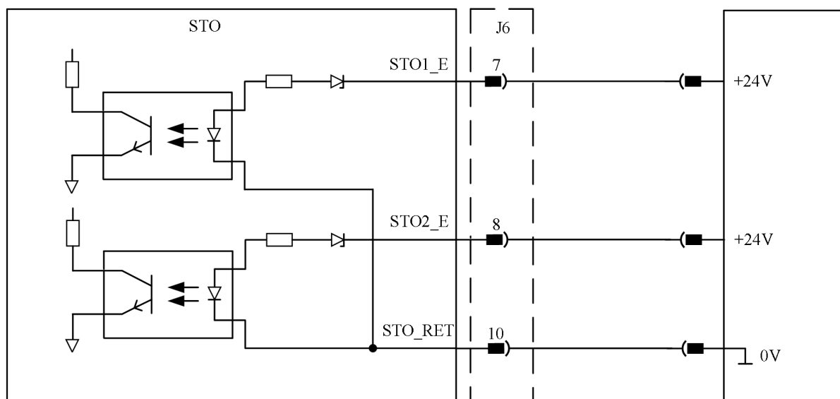
图 8-16 STO 接线示意图
