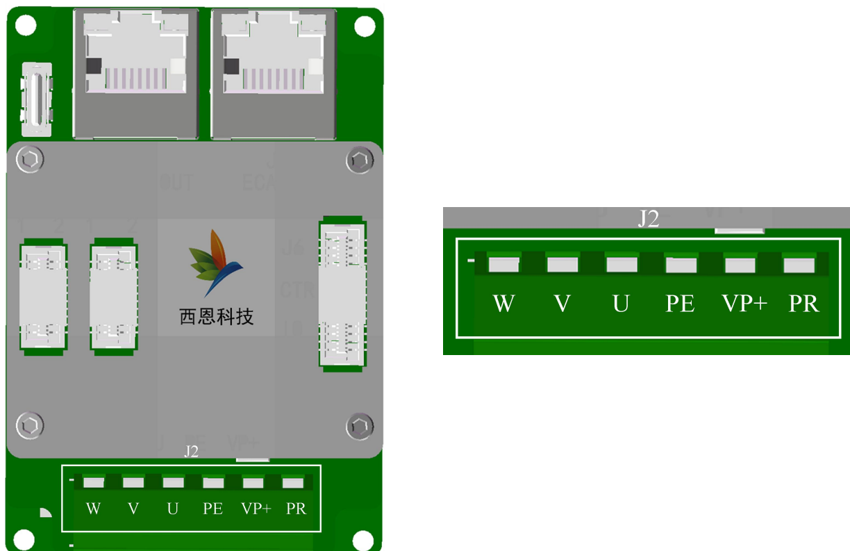
图 4-4 动力线接口示意图
