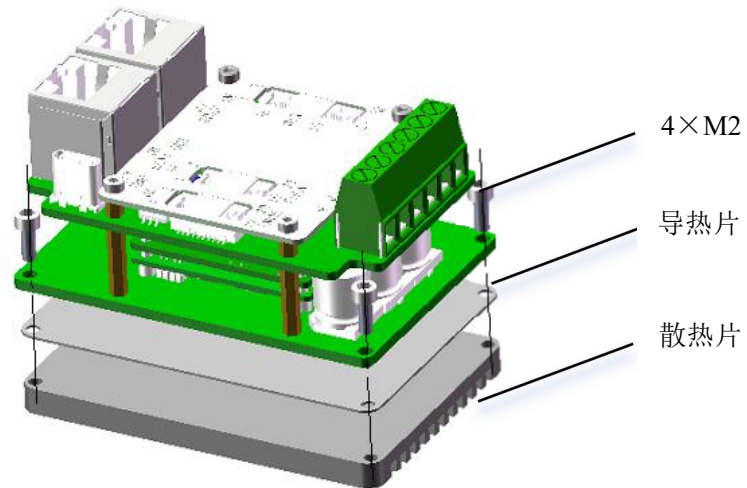
图 3-1 散热附件安装示意图
