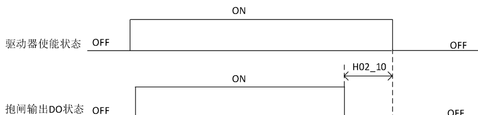
图 8-18 抱闸输出时序图
