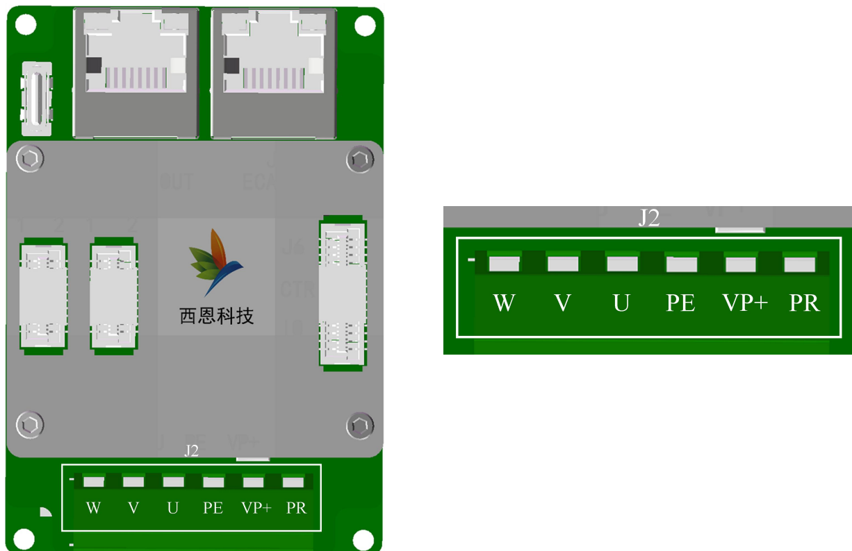
图 4-2 电源接口示意图
