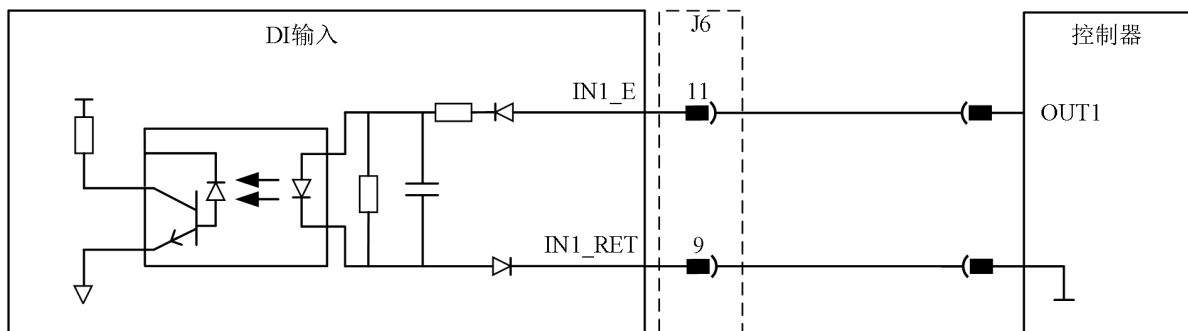
图 4-12 高速 DI 接线示意图
