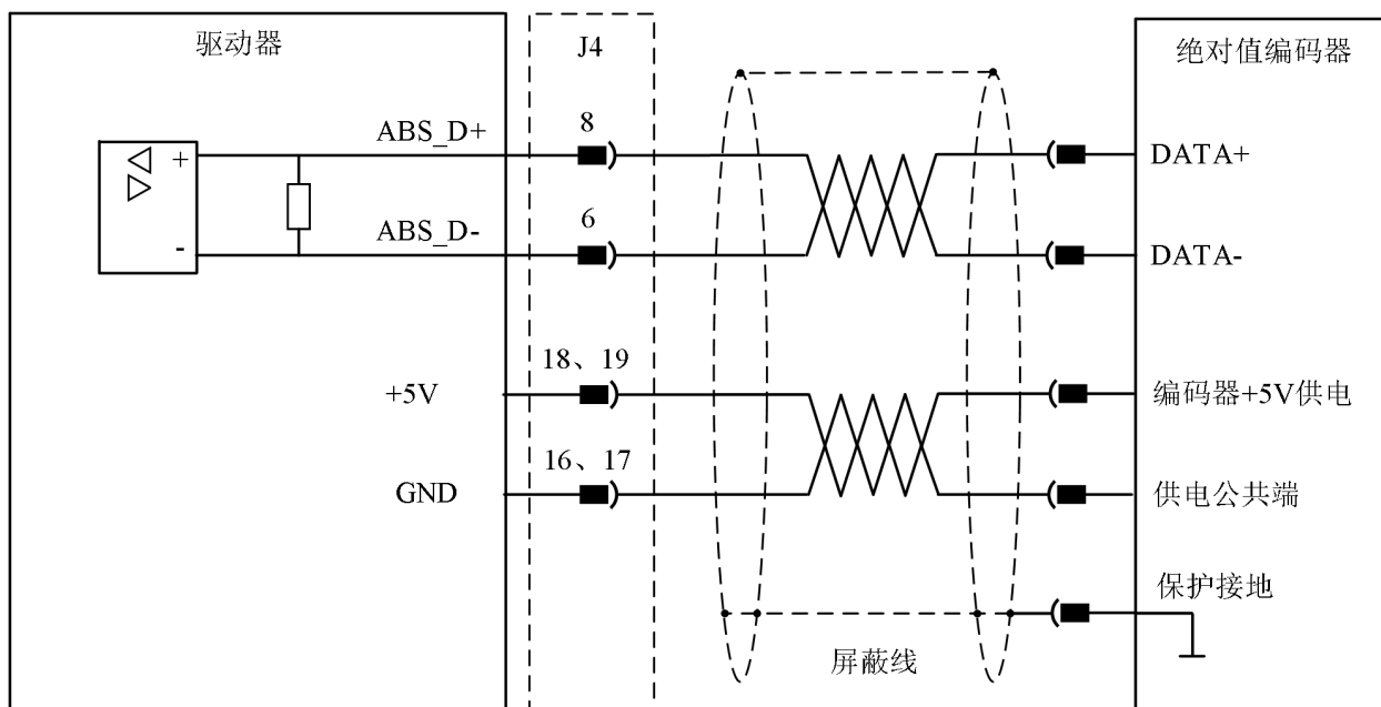
图 4-26 不带时钟信号 BiSS-C/SSI 编码器接线示意图
