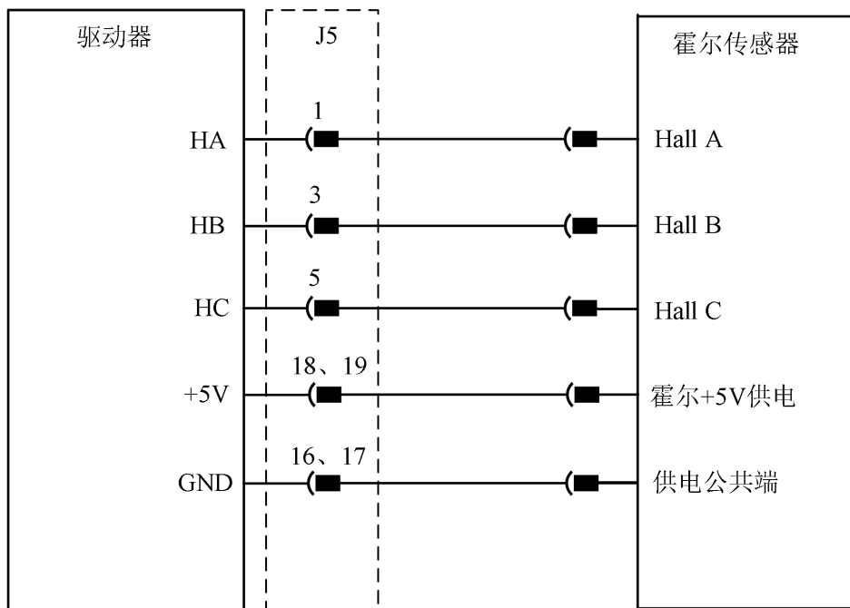
图 4-28 单霍尔接线示意图
