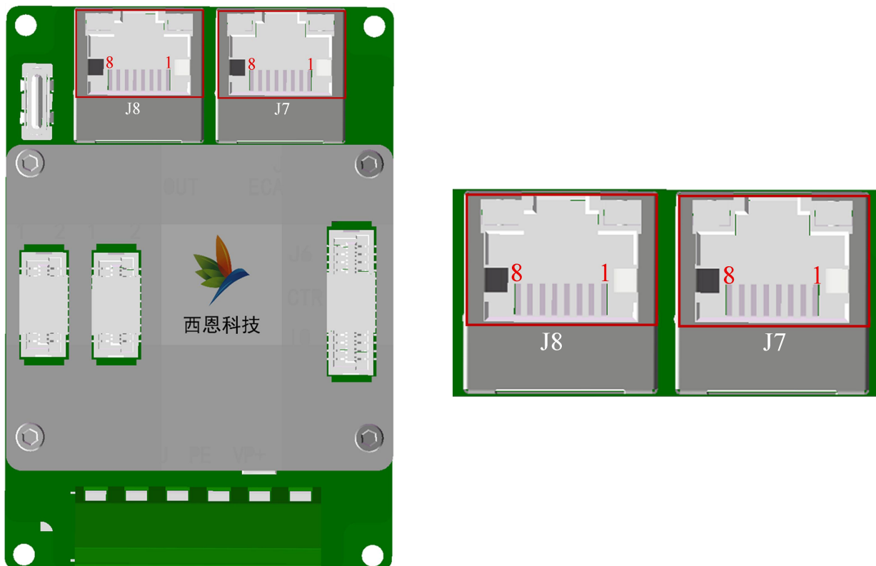
图 4-9 EtherCAT 通讯接口示意图
