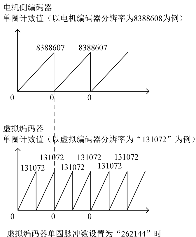
图 1-7 虚拟编码器单圈脉冲数不同配置下计数周期对比示意图
