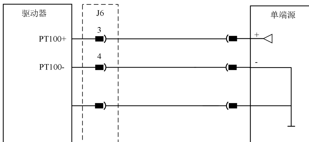
图 4-21 模拟量 2（PT100）接线示意图
