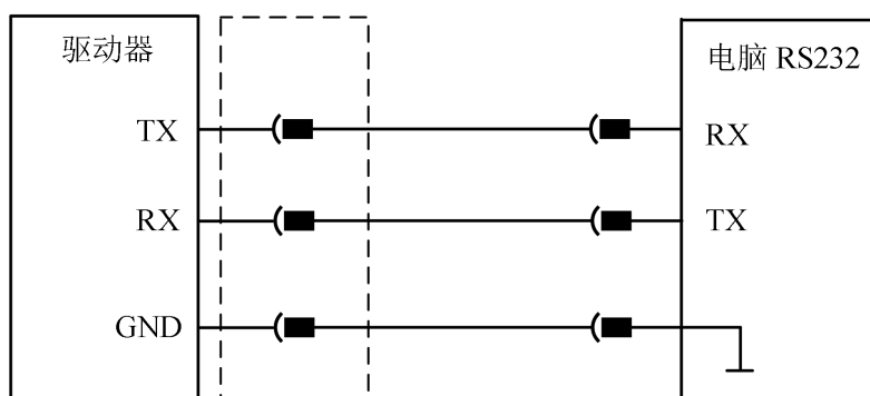
图 8-15 RS232 接线示意图
