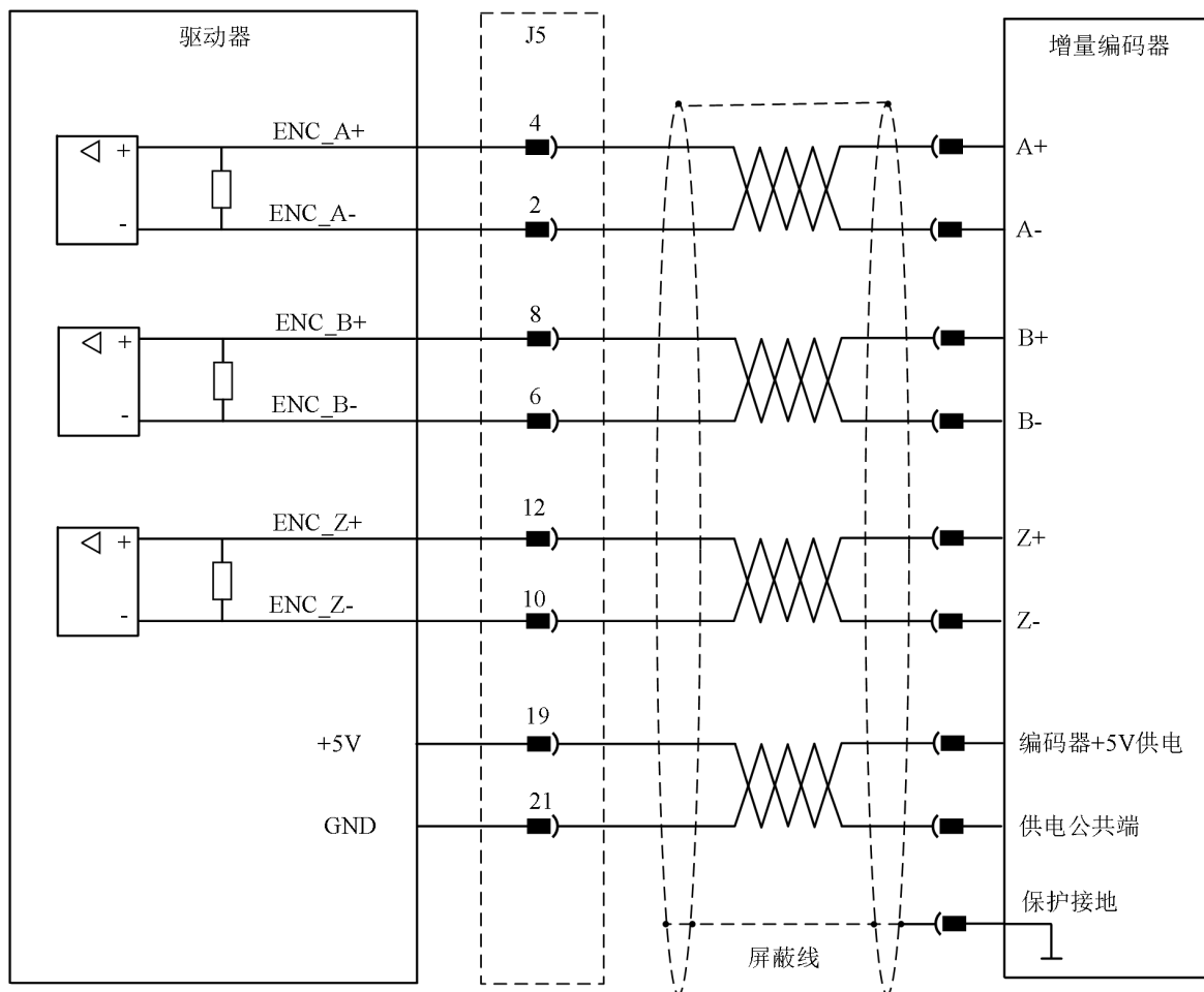
图 4-25 增量编码器接线示意图
