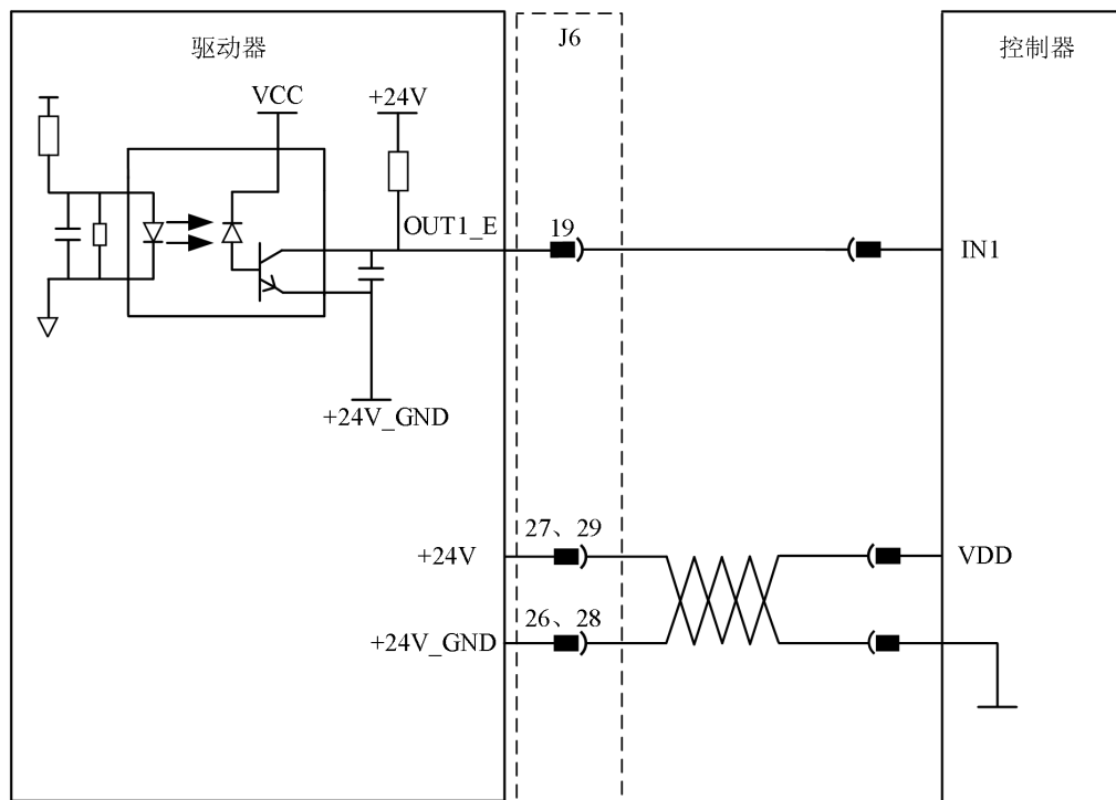
图 4-15 源型输出接线图
