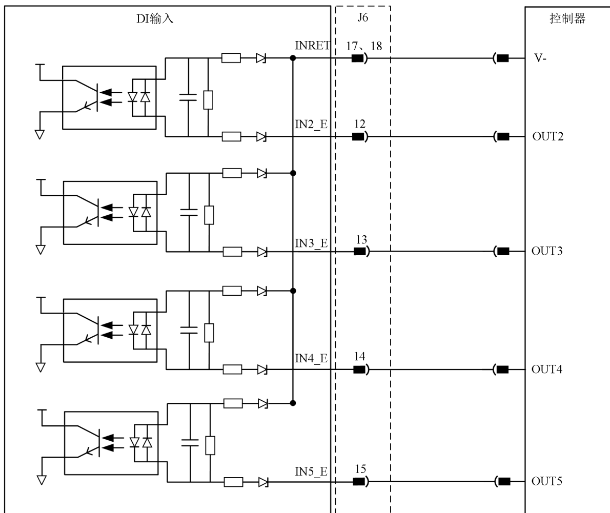
图 4-14 源型输入接线图
