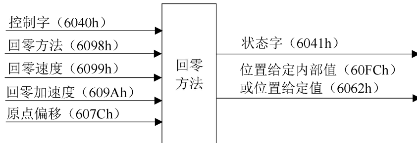
图 9-12 回零模式（HM）控制框图
