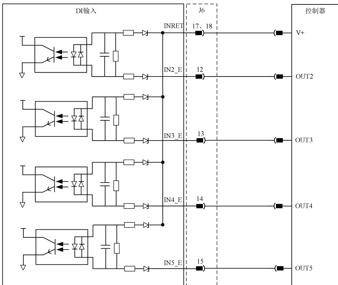
图 4-13 漏型输入接线图
