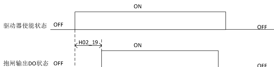
图 8-19 抱闸输出时序图
